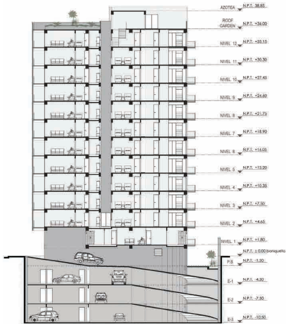
CORTE LONGITUDINAL
