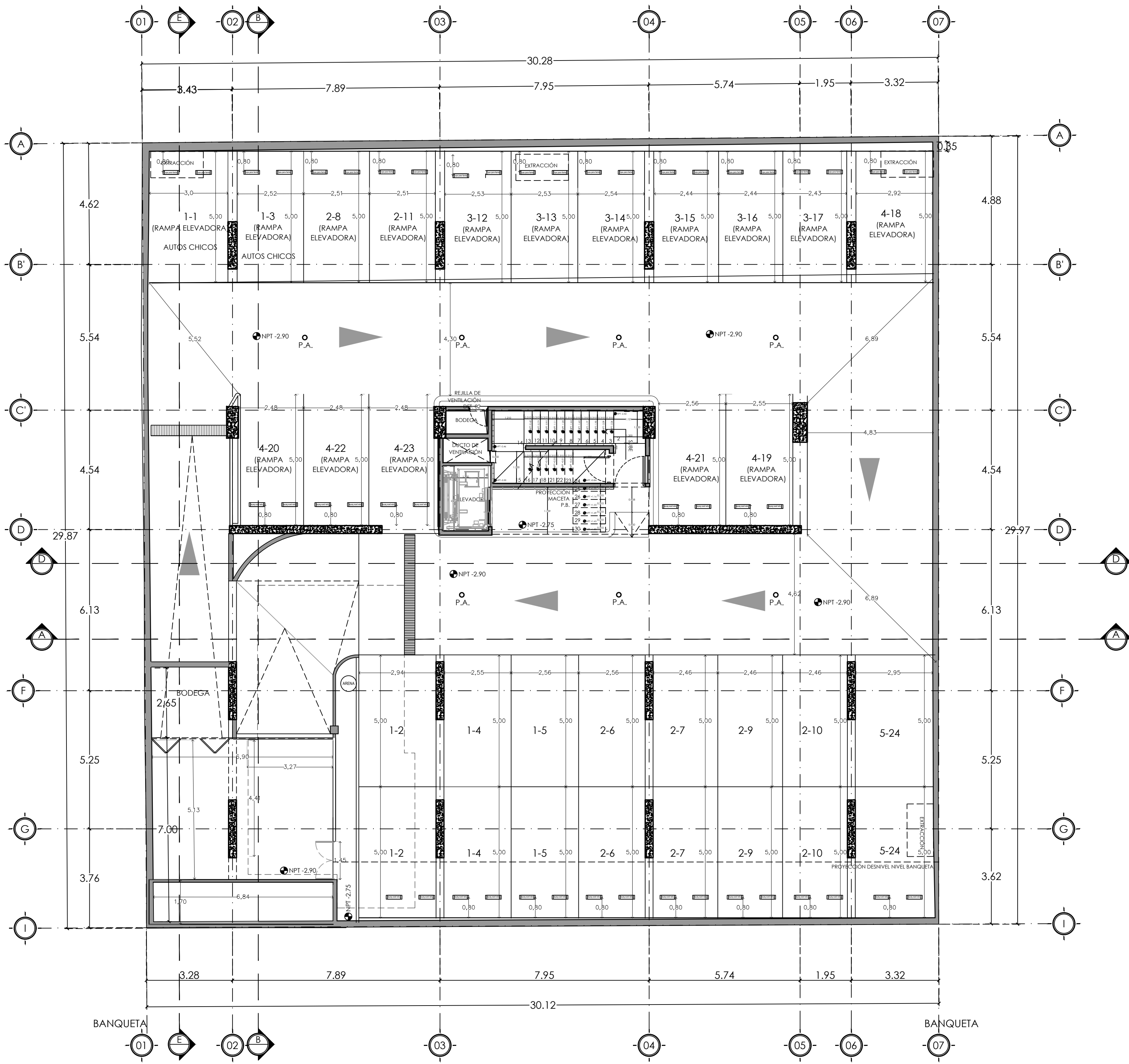
PLANTA SÓTANO ESCALA 1:100
