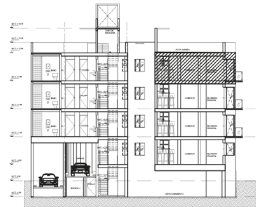
CORTE ESQUEMATICO
