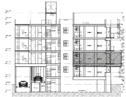
CORTE ESQUEMATICO
