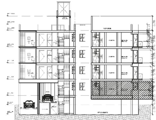
CORTE ESQUEMATICO
