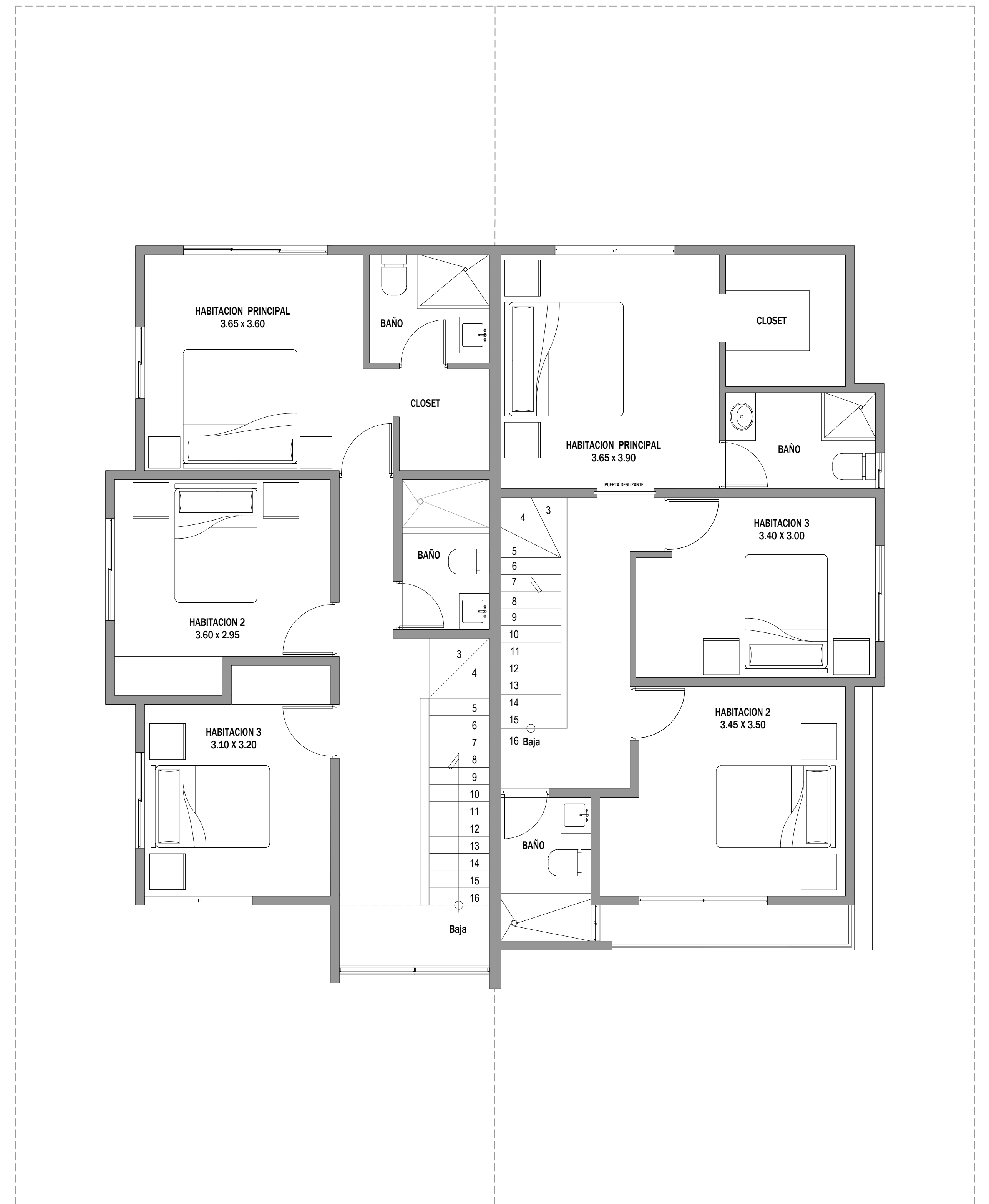
1 PLANTA ARQUITECTONICA AMUEBLADA 2DO NIVEL A.3 VILLA TOULOUSE - TIPO B / C
