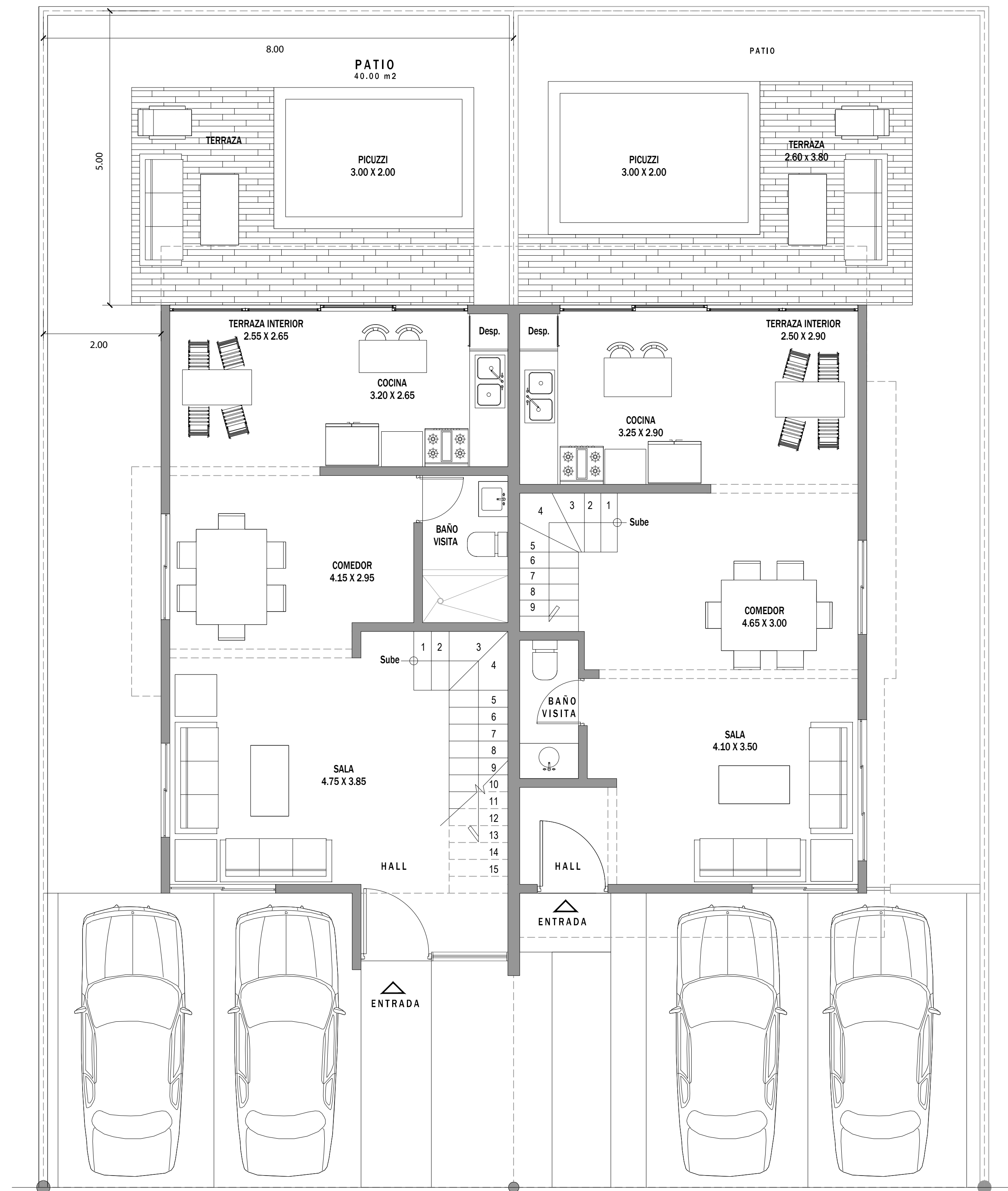
1 PLANTA ARQUITECTONICA AMUEBLADA 1ER NIVEL A.2 VILLA TOULOUSE - TIPO B / C
