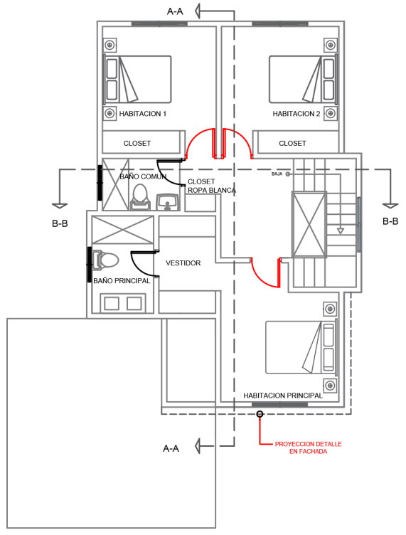
PLANTA ARQUITECTONICA DEL 2DO NIVEL
