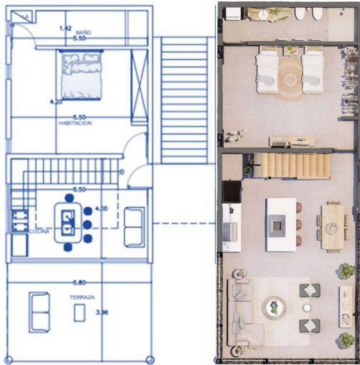
PLANTA ARQUITECTONICA SEGUNDO NIVEL
