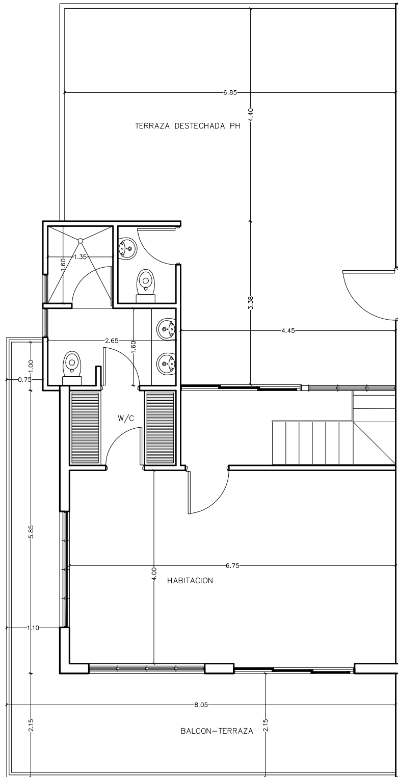
PLANTA DIMENSIONADA 2DO NIVEL DE PENT-HOUSE
