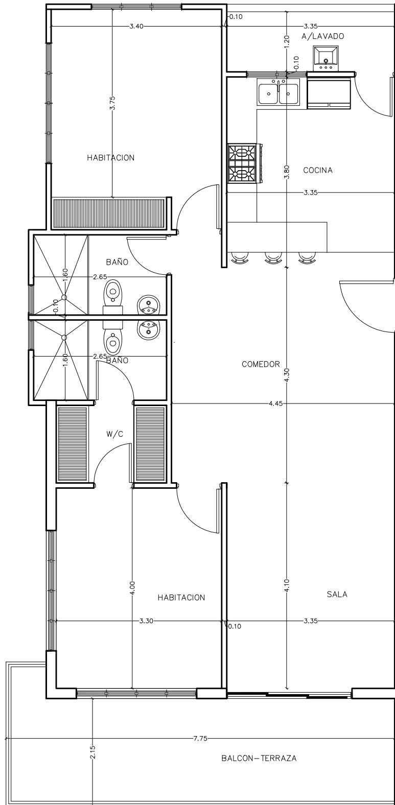
PLANTA DIMENSIONADA APART. TIPO 2 HABITACIONES
