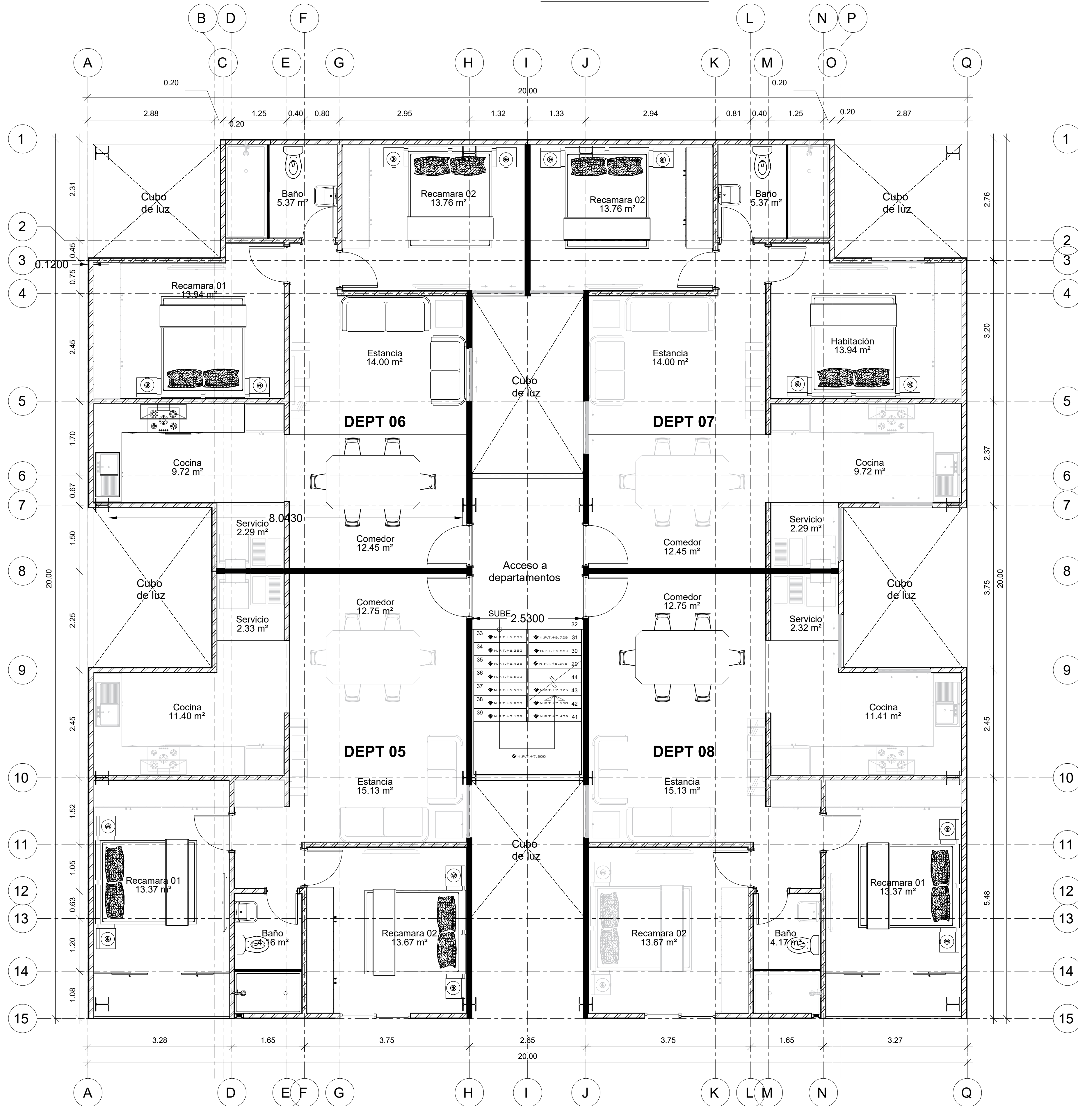
1 PLANTA 2do NIVEL ARQ-05 EDIFICIO DEPARTAMENTOS ESC:1:50
