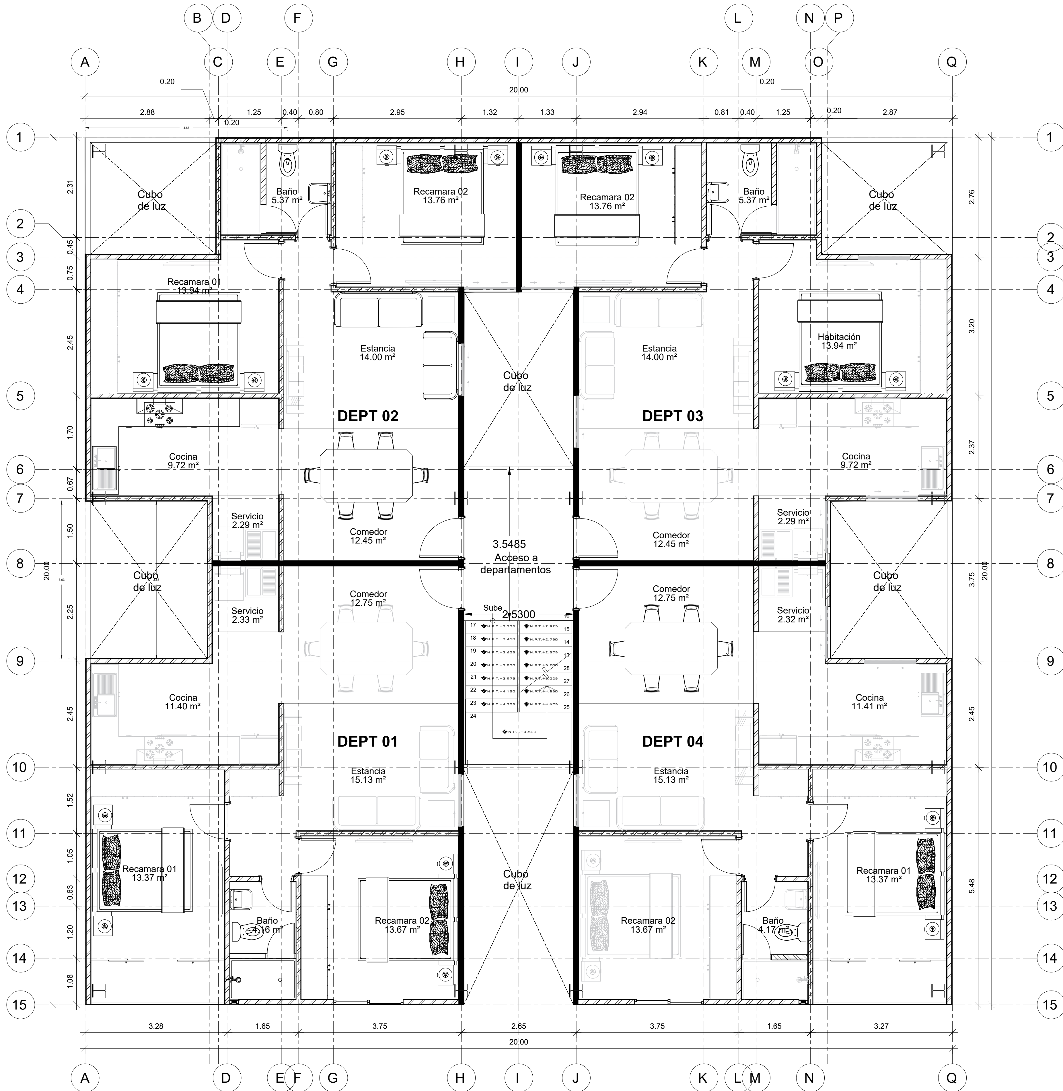
1 PLANTA 1er NIVEL ARQ-04 EDIFICIO DEPARTAMENTOS ESC:1:50
