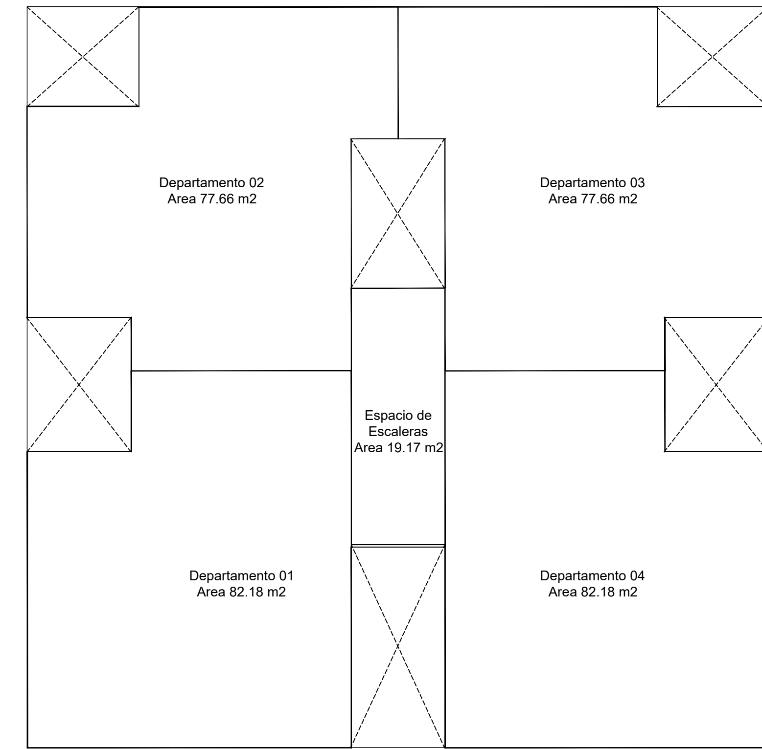
2 PLANTA DEPARTAMENTOS ARQ-04 EDIFICIO DEPARTAMENTOS SIN ESCALA
