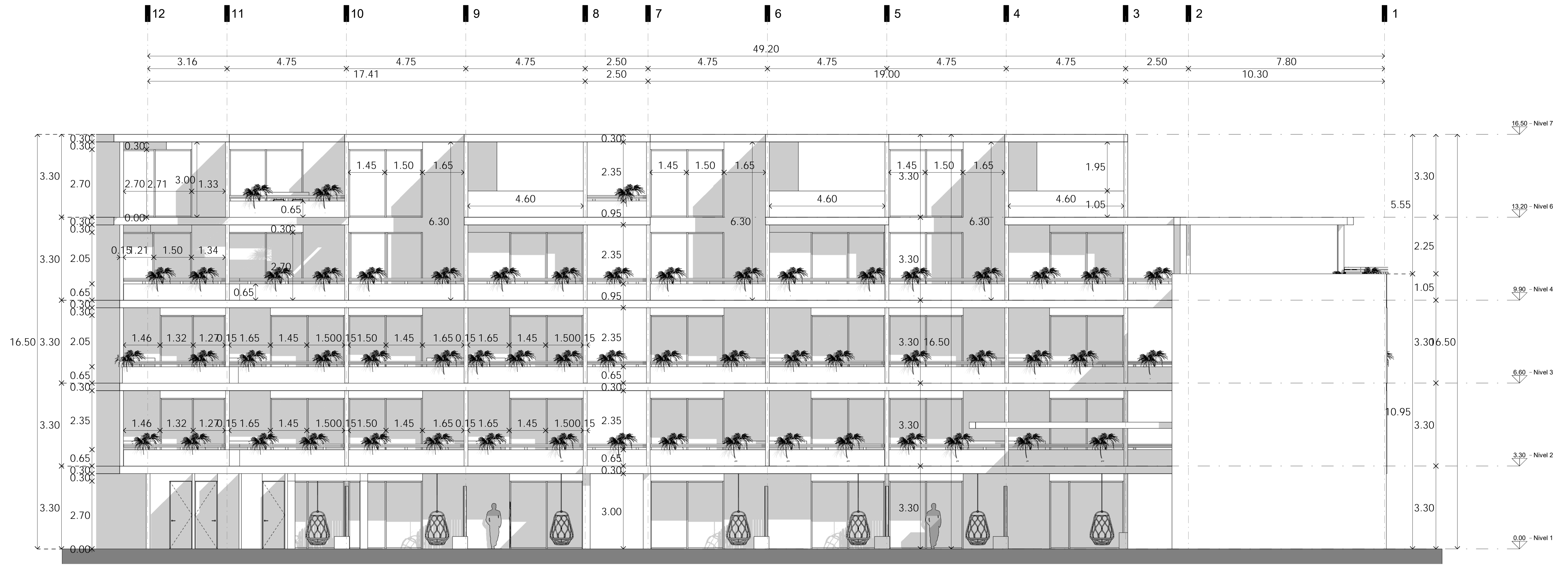
1 FACHADA LATERAL 1:75
