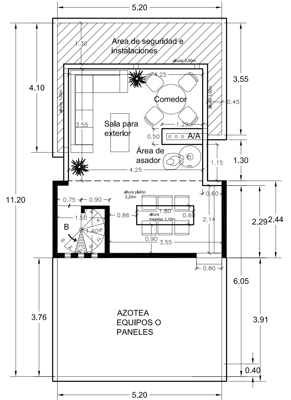
PLANTA AZOTEA
