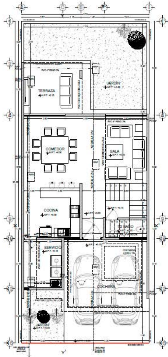
PLANTA BAJA
