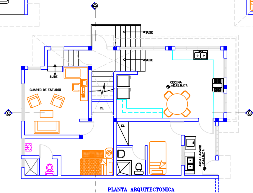
PLANTA ARQUITECTONICA
