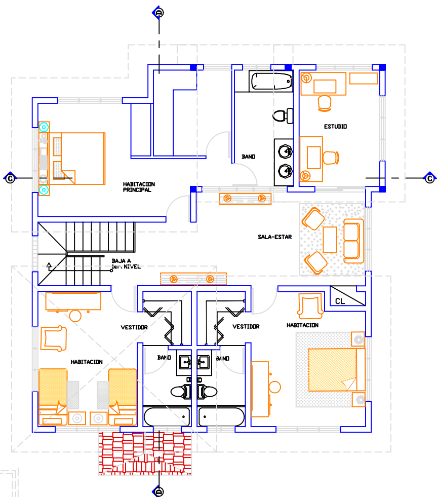
PLANTA ARQUITECTONICA SEGUNDO NIVEL ESC. 1:50
