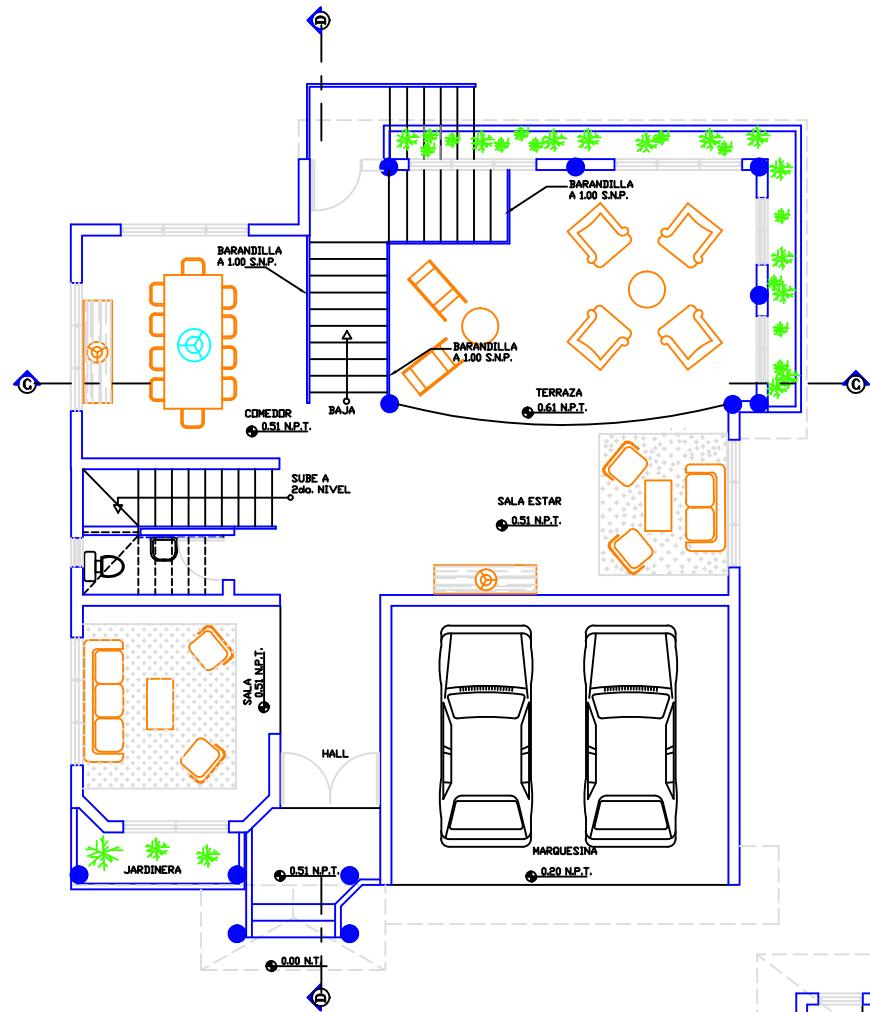
PLANTA ARQUITECTONICA PRIMER NIVEL ESC. 1:50
