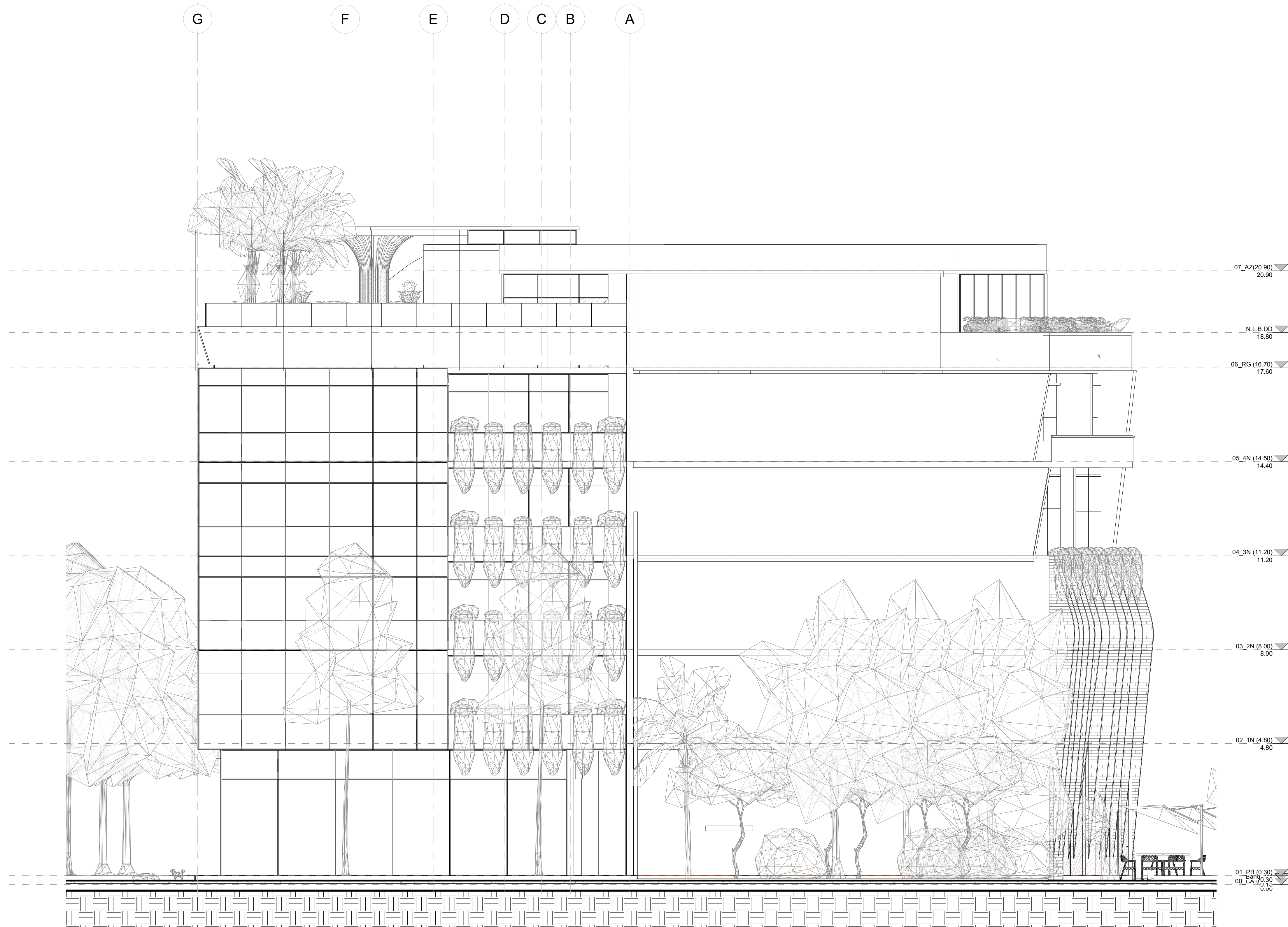
1 Fachada Lateral Derecha 1 : 75
