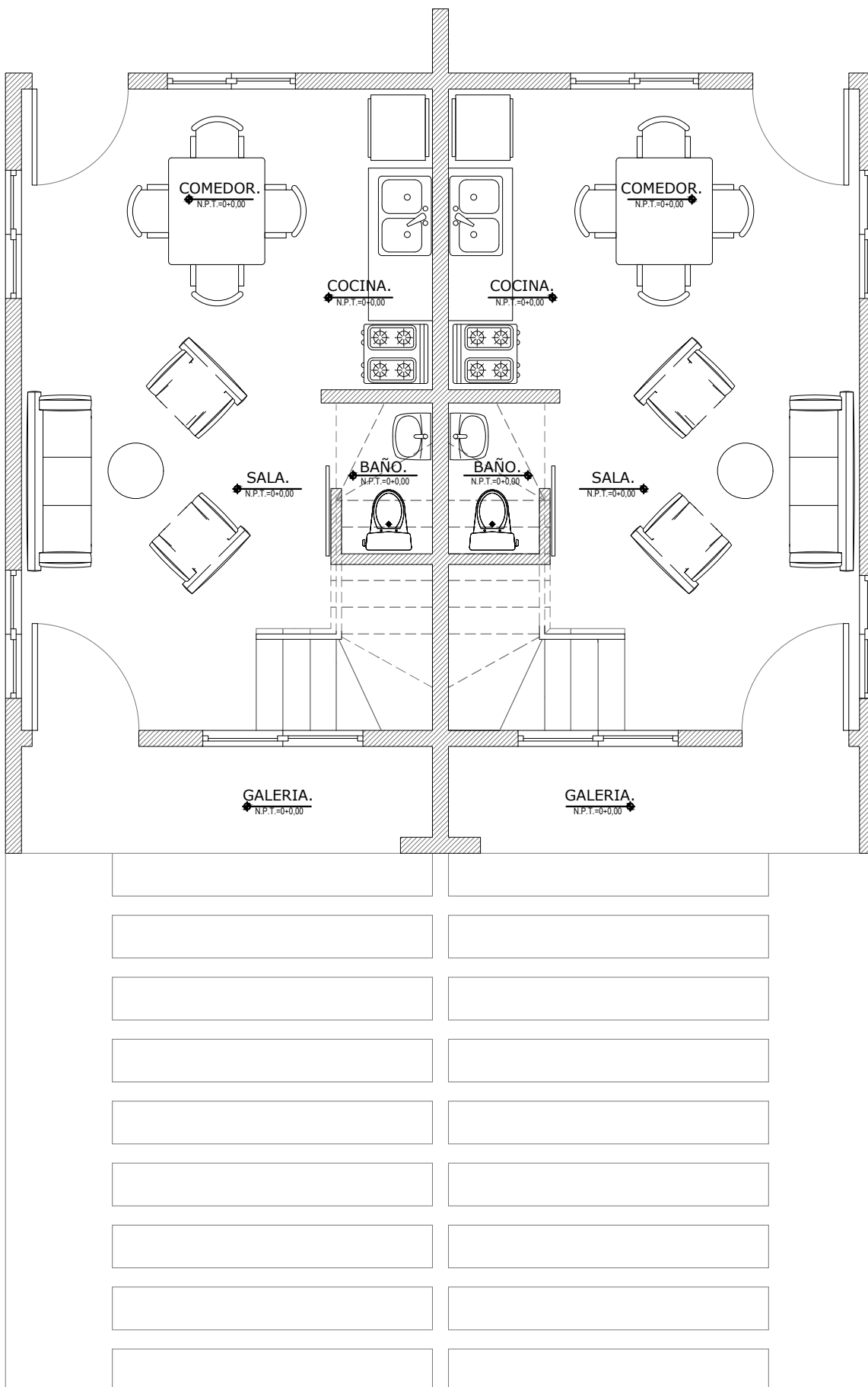
Planta Arquitectonica. 1er. Nivel. Esc. 1:50
