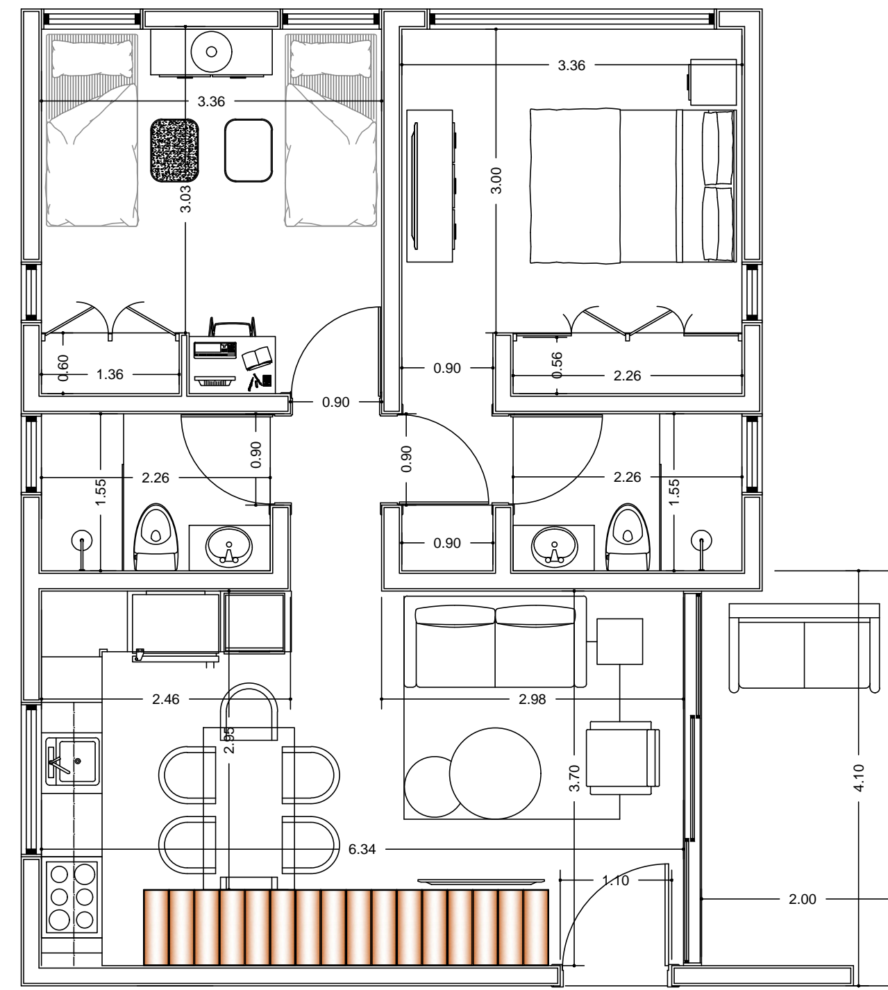
Tipologia #3 Bloque A-B Escala N/A
