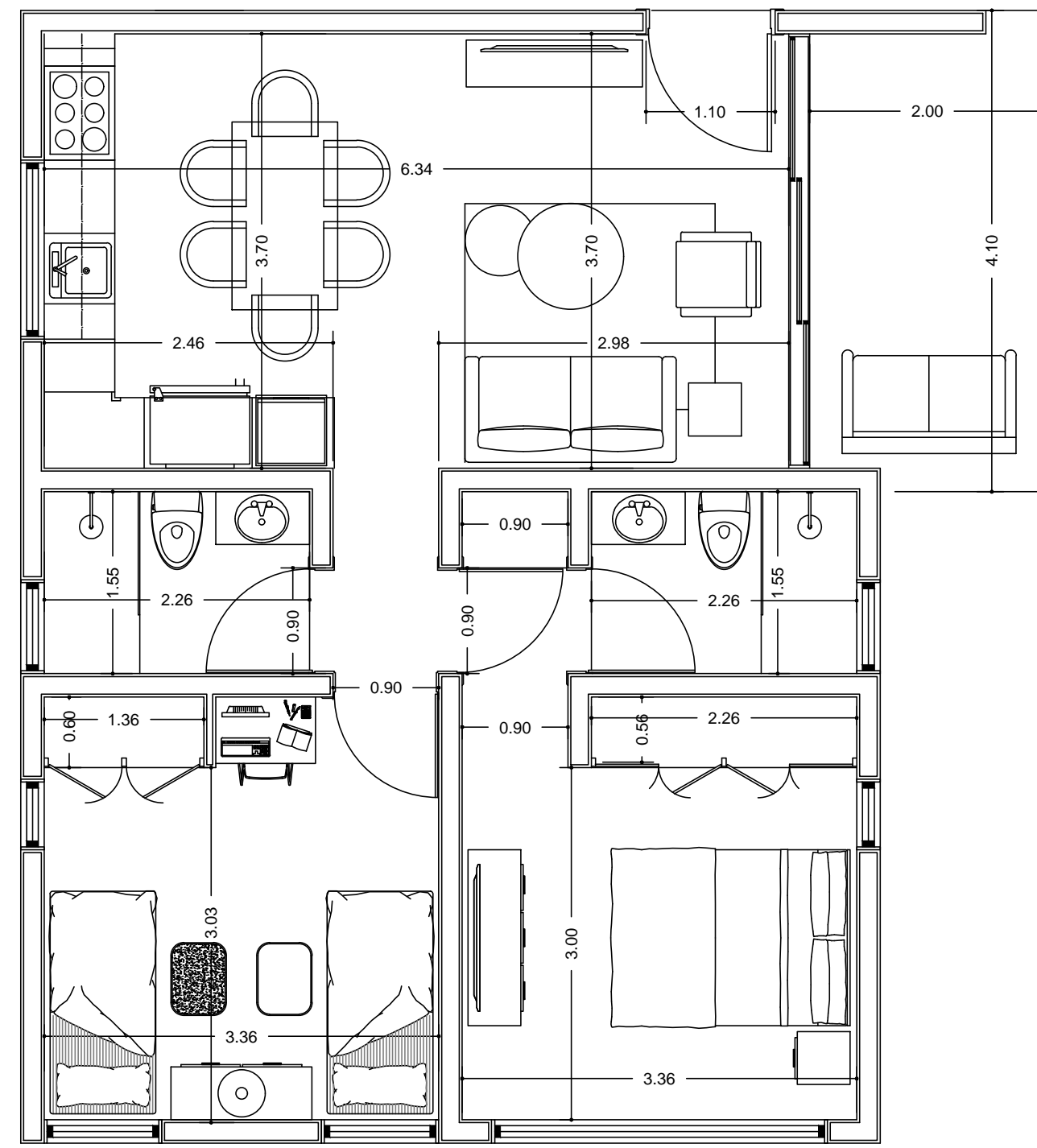
Tipologia #1 Bloque A-B Escala N/A
