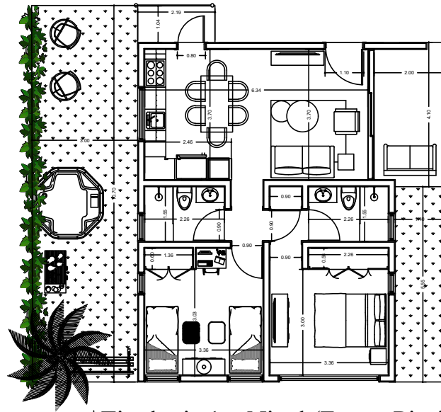
Tipologia 1er Nivel (Frente Piscina)
