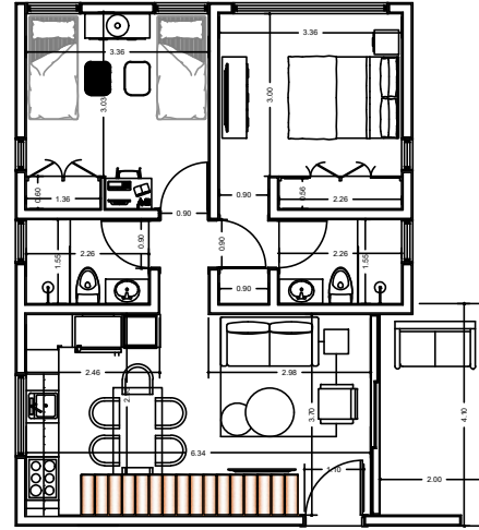
Tipologia 3er Nivel
