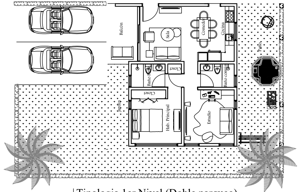
Tipologia 1er Nivel (Doble parqueo)
