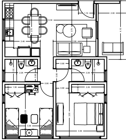
Tipologia 2do Nivel
