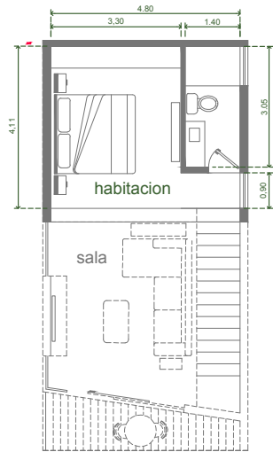
planta alta loft
