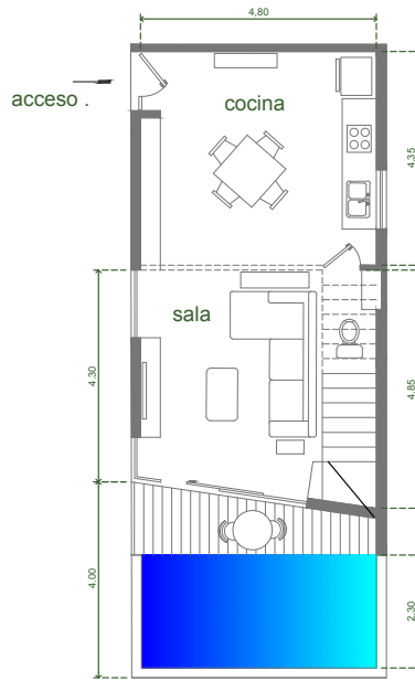
planta baja loft
