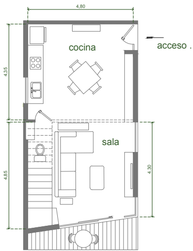
planta baja loft
