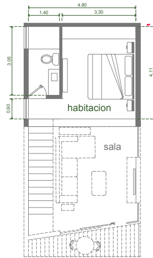
planta alta loft
