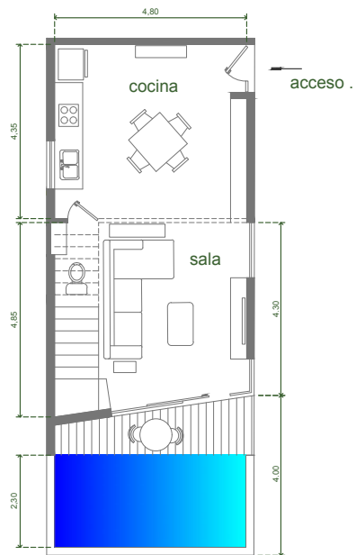
planta baja loft
