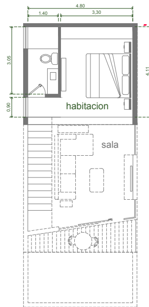
planta alta loft
