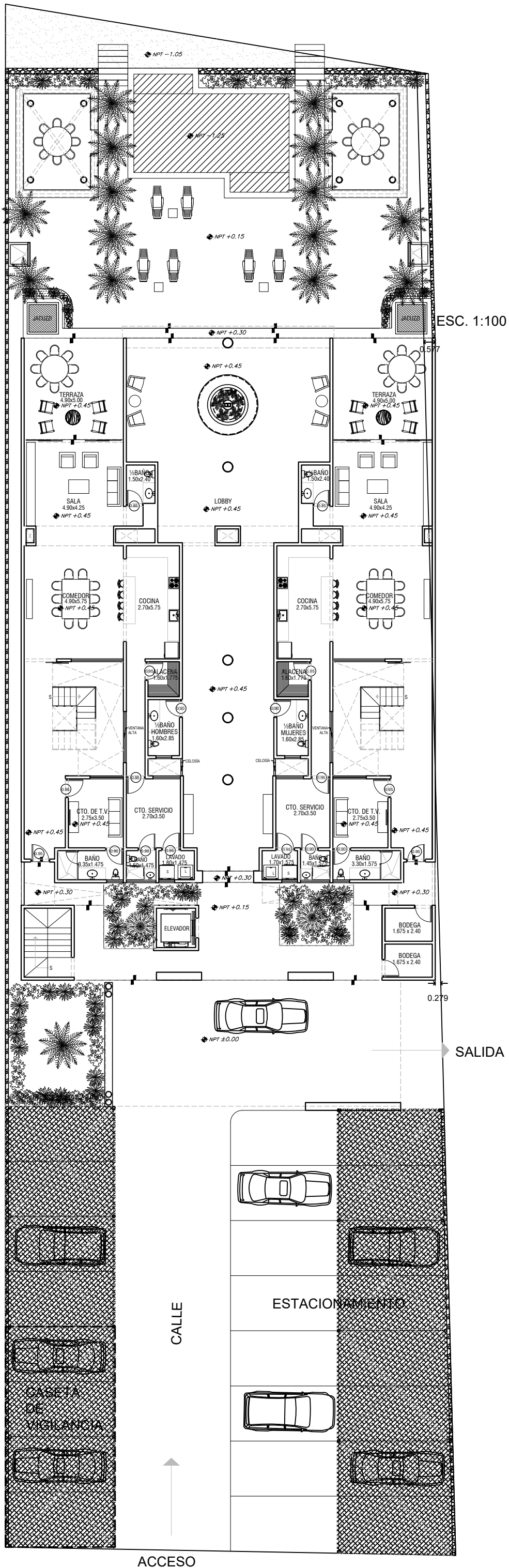
PLANTA BAJA
