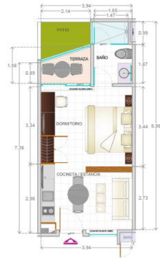
PLANTA TIPO 2A
