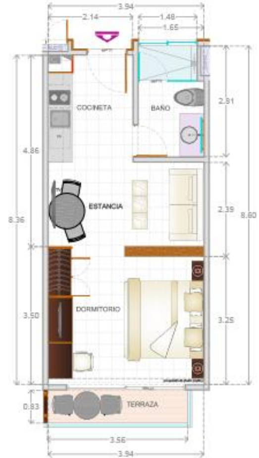
PLANTA TIPO 4A
