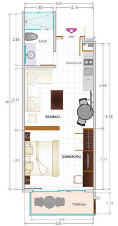
PLANTA TIPO 3A
