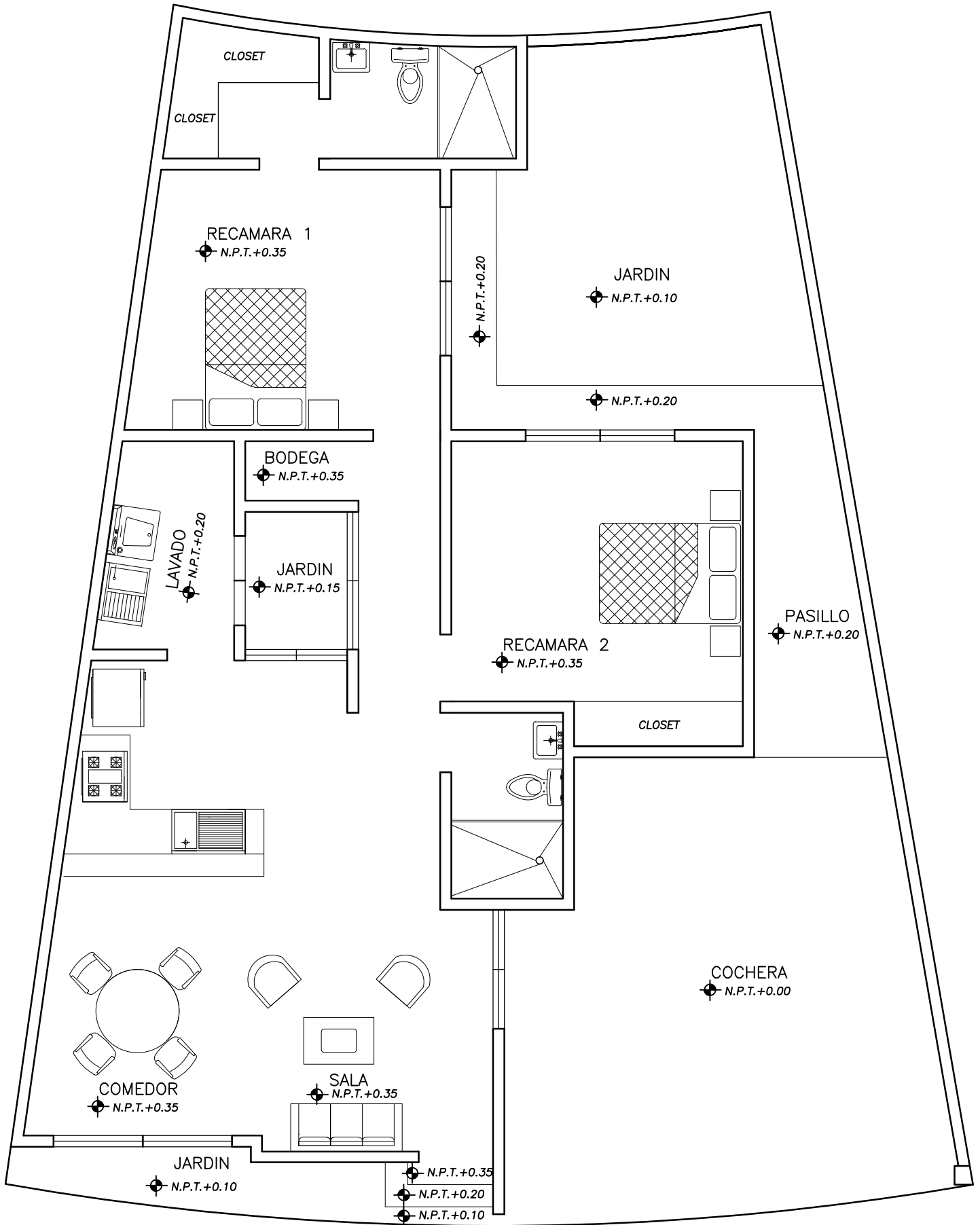
PLANTA ARQUITECTONICA SUP= 98.00 m2
