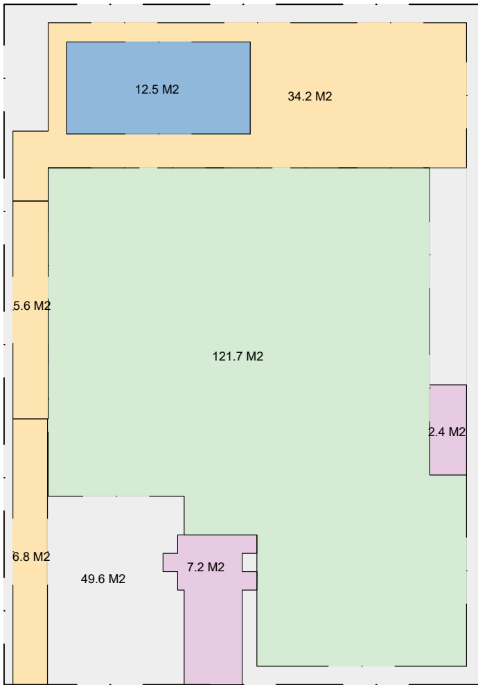
PRIMER NIVEL
