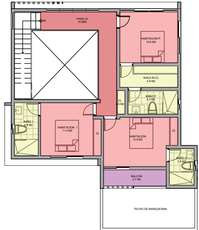
SEGUNDO NIVEL
