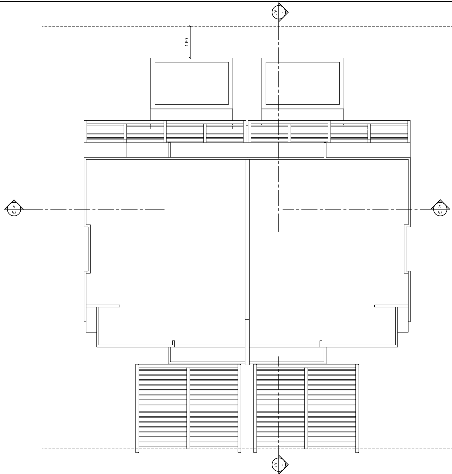
1 PLANTA ARQUITECTONICA DIMENSIONADA 1ER NIVEL A.2 VILLA TOULOUSE - TIPO A ESCALA 1:40
