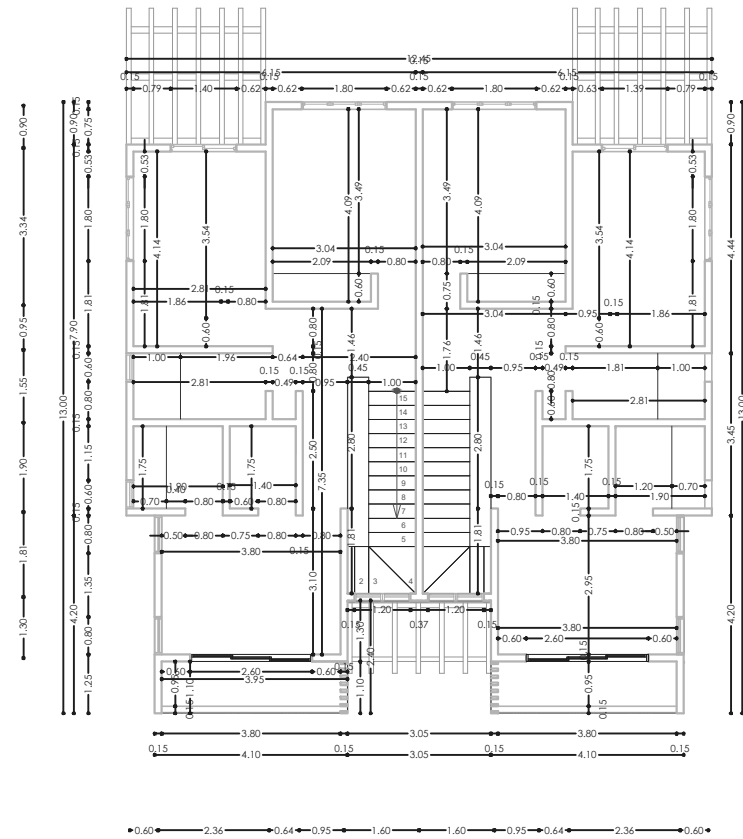
PLANTA DIMENSIONADA NIVEL 2 ESC.: N/A
