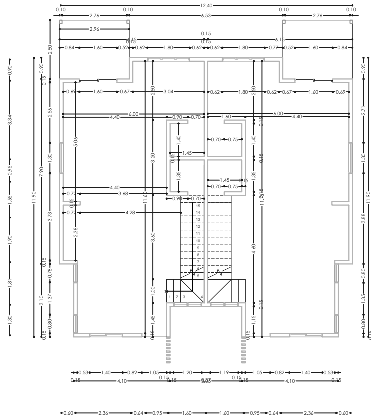
PLANTA DIMENSIONADA NIVEL 1 ESC.: N/A
