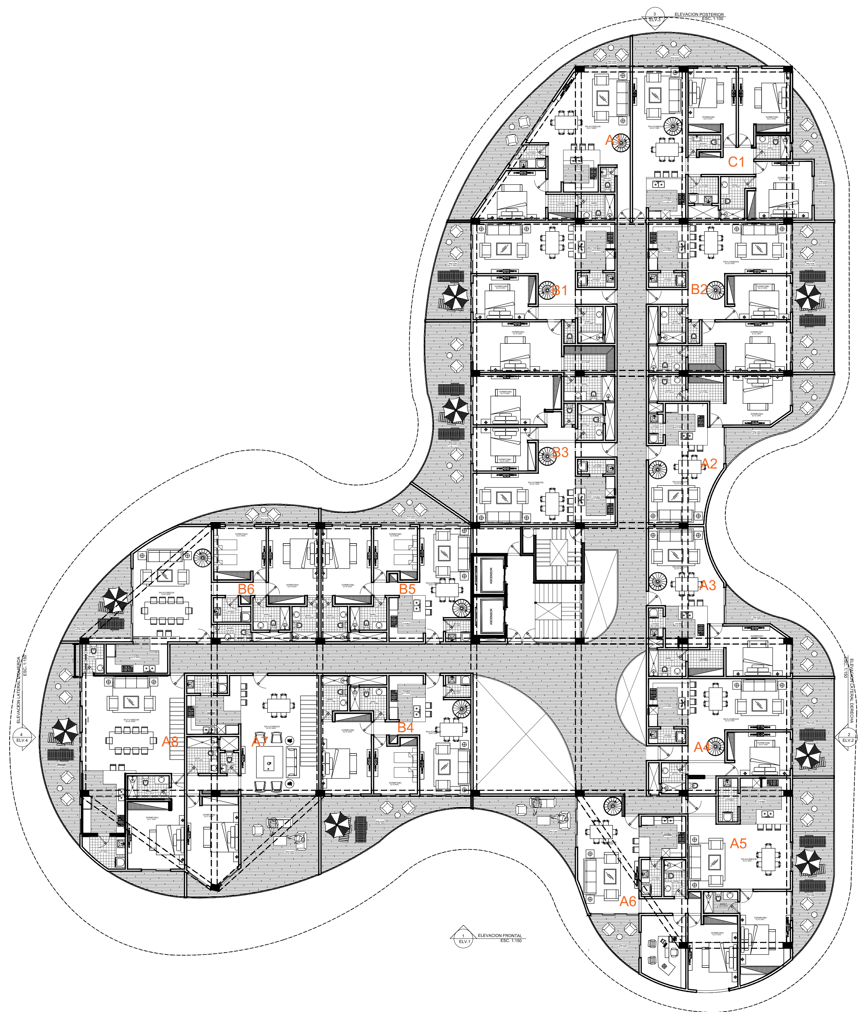
ARQ.#1 NIVEL.0 PLANTA ARQ. 4TO NIVEL 4-NIVELES ESC. 1:150
