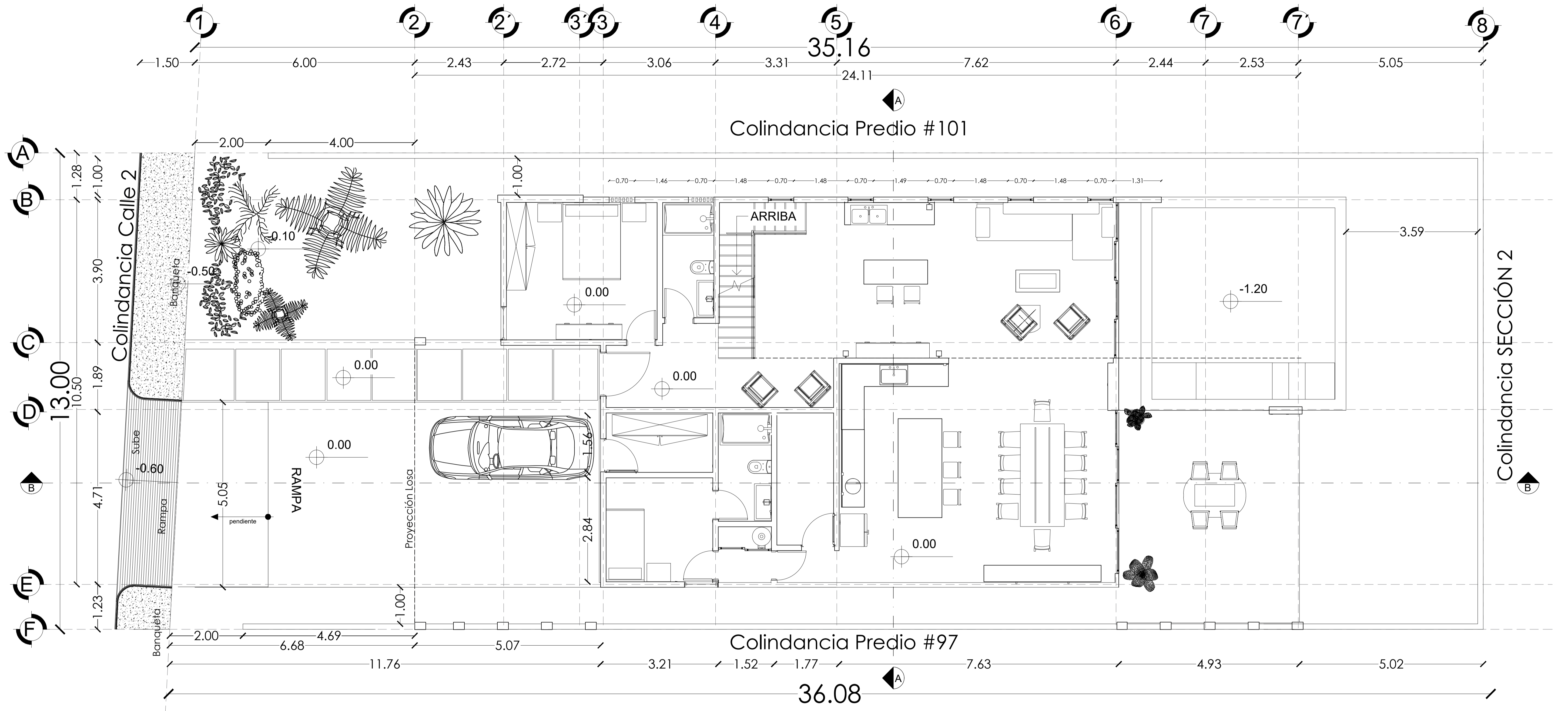
PLANTA BAJA
