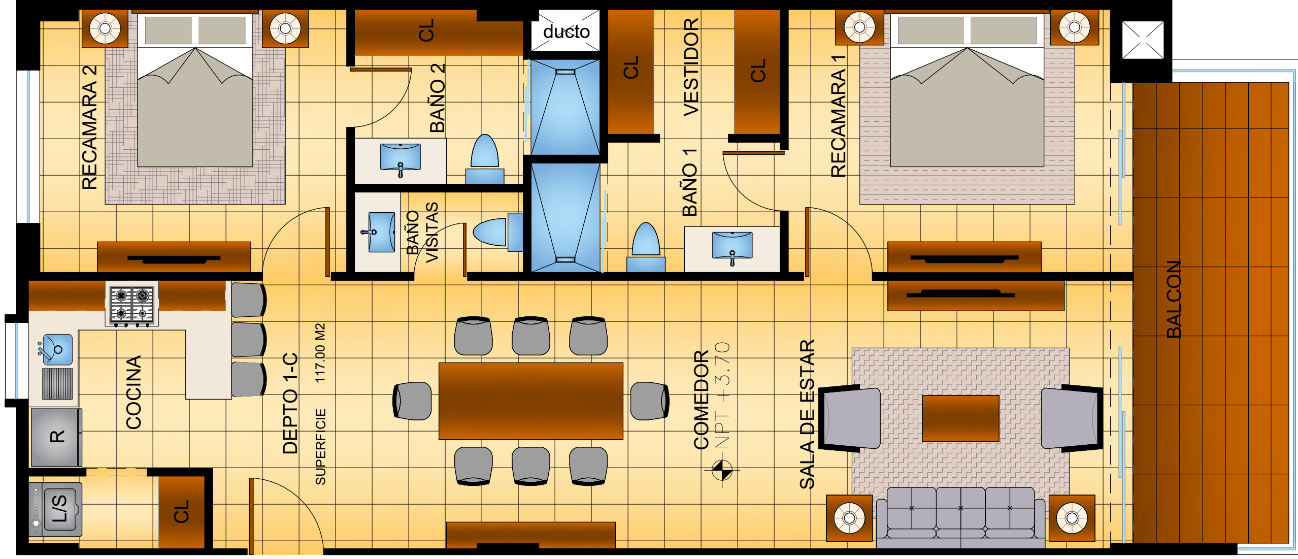
PLANTA ARQUITECTONICA DEPARTAMENTO TIPO 1 ESCALA 1:50
