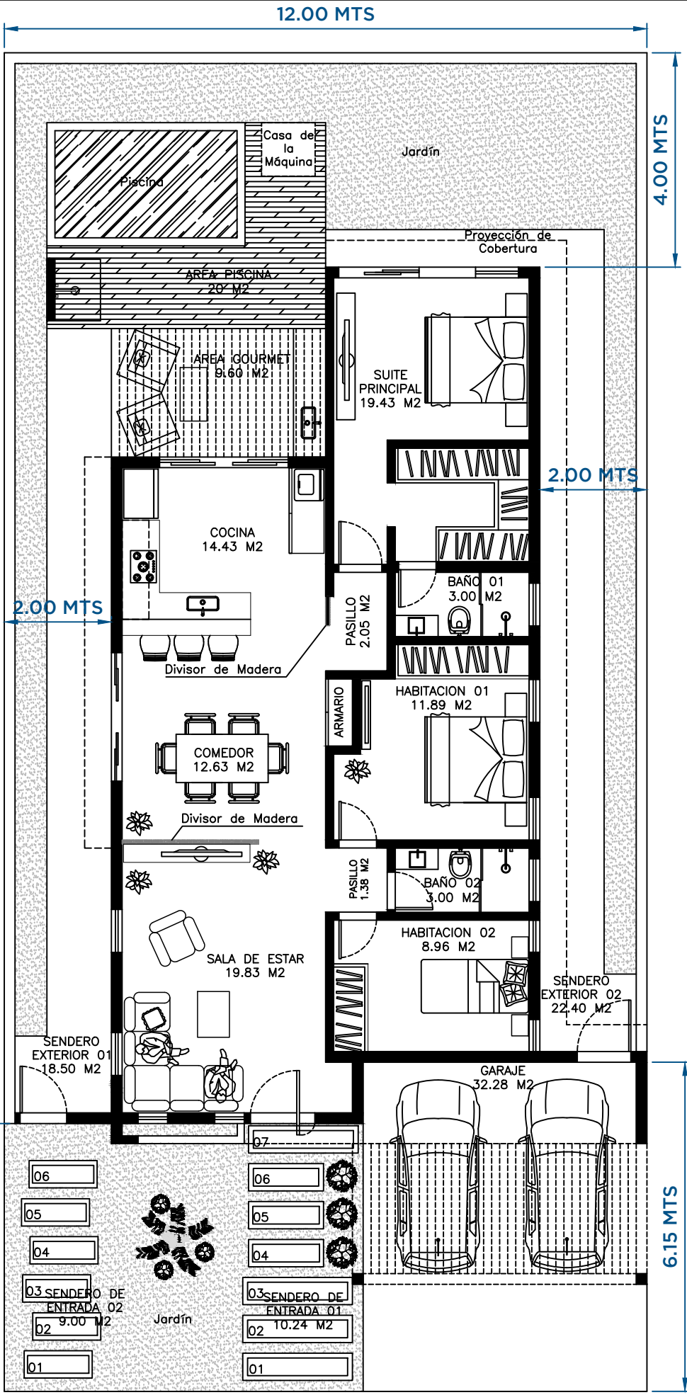
Planta de Diseño Escala - 1:100
