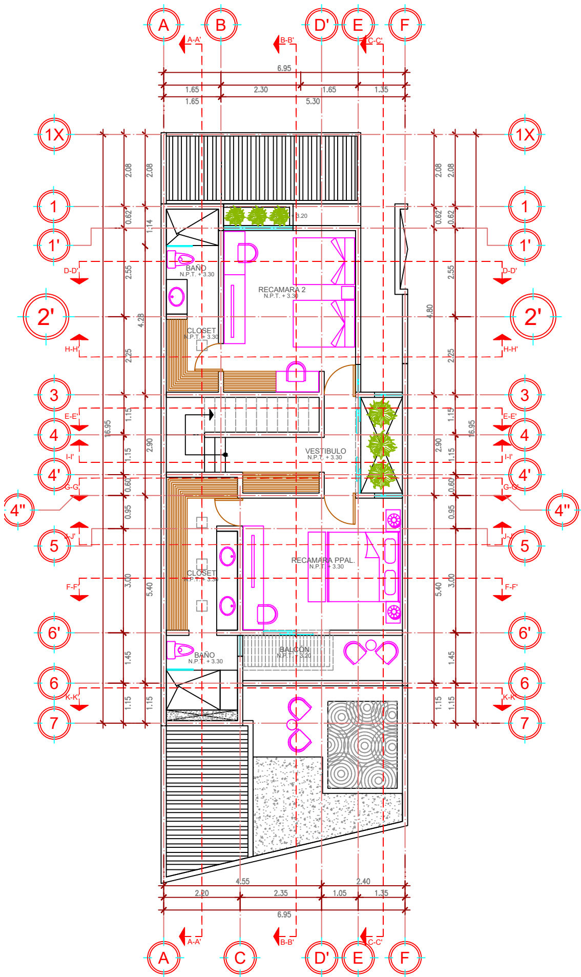
PLANTA ALTA
