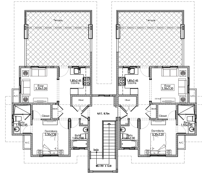
PLANTA ARQ. 4TO NIVEL
