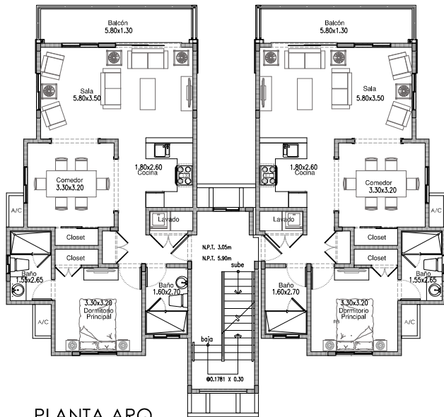
PLANTA ARQ. 2DO-3ER NIVEL
