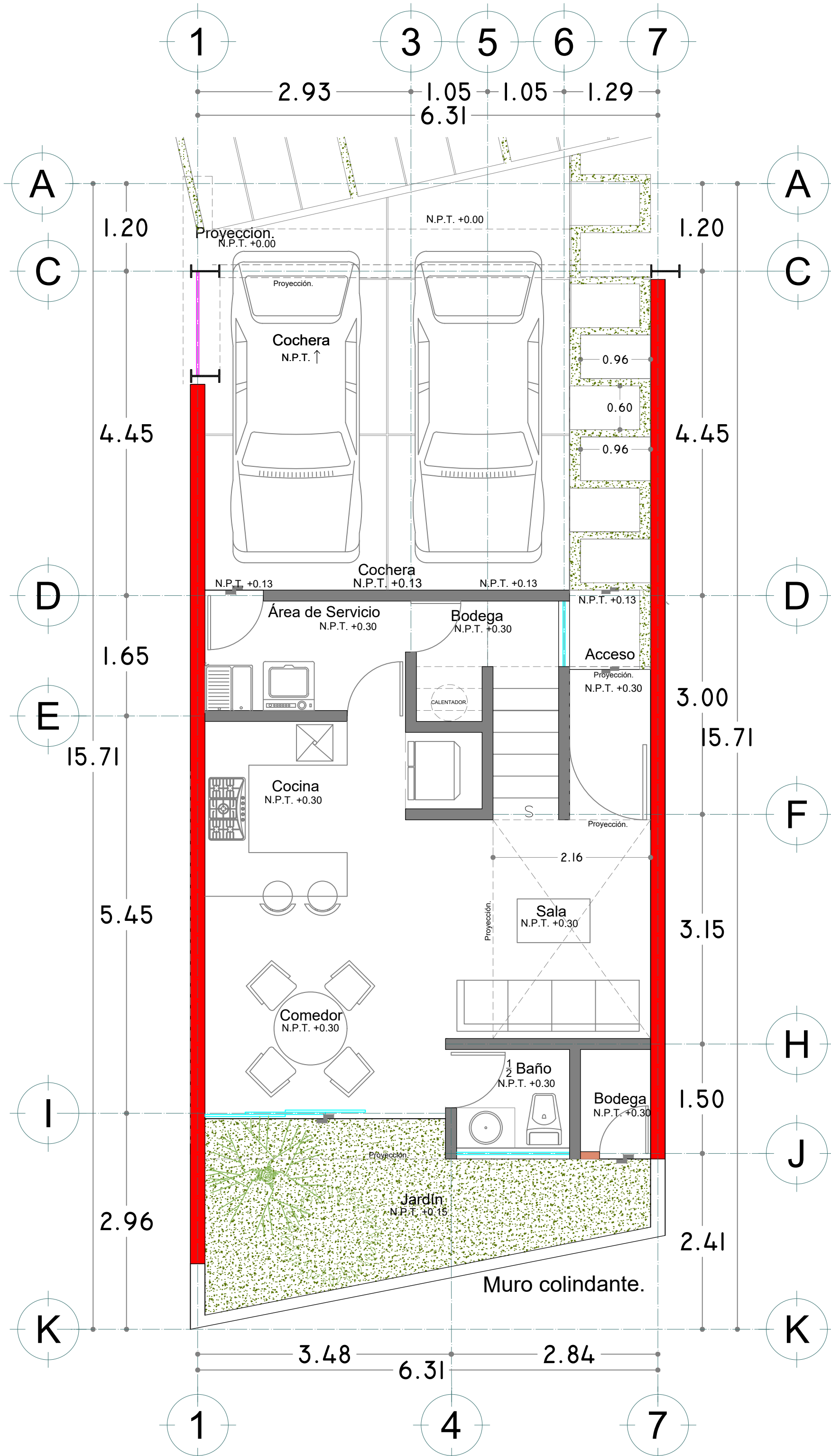
PLANTA DE CONJUNTO | BAJA
