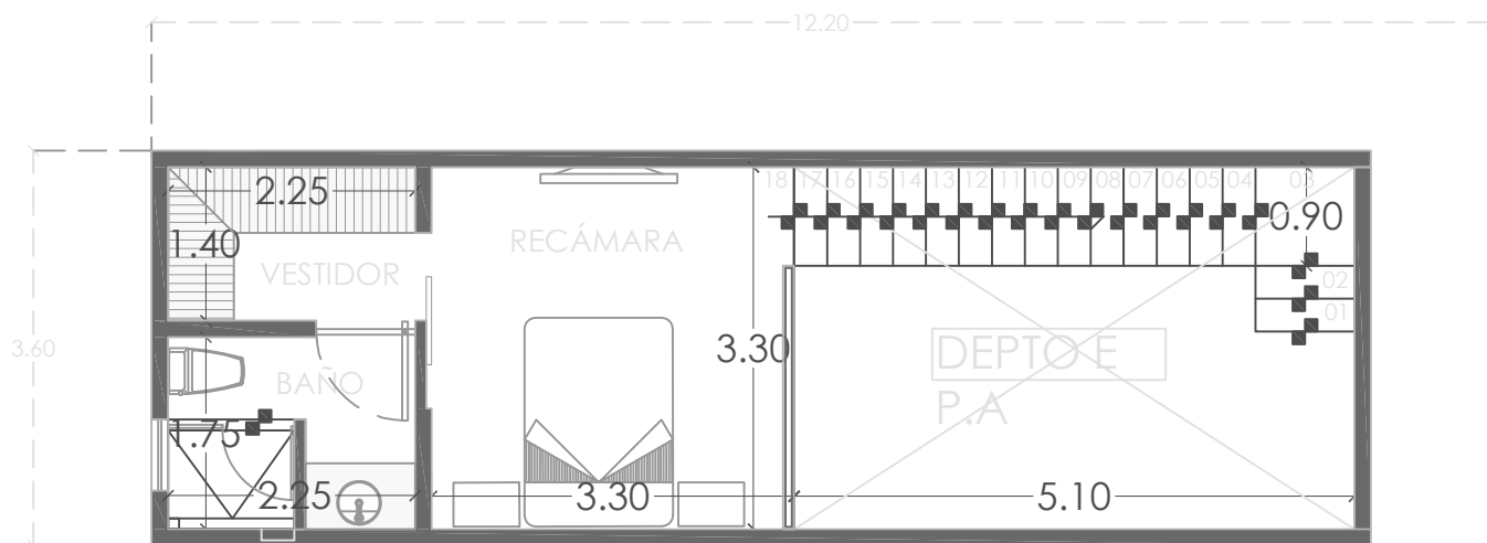
PLANTA ALTA
