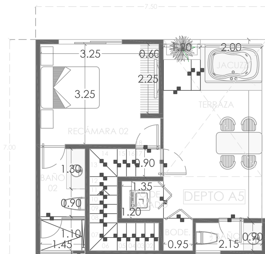
PLANTA ALTA
