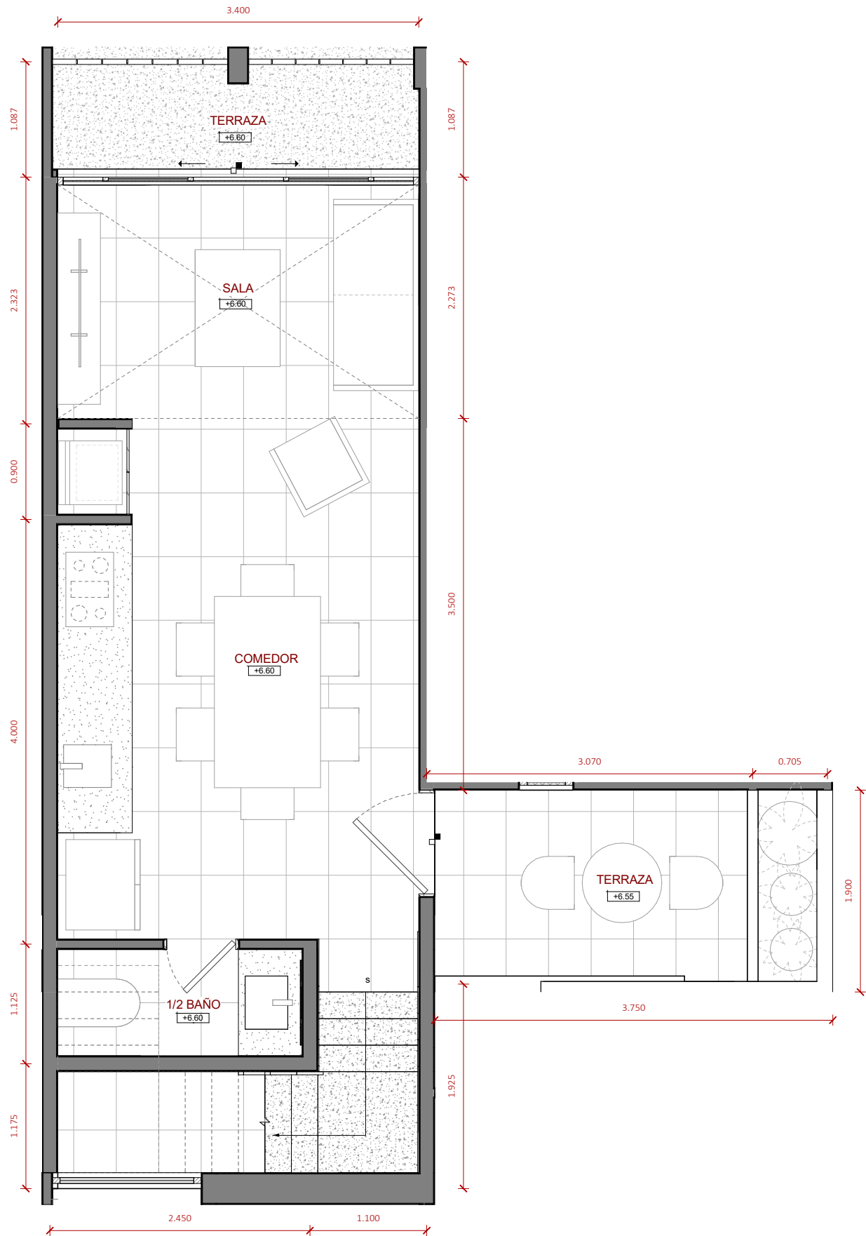
NIVEL 3 +6.60 ESCALA 1 : 50
