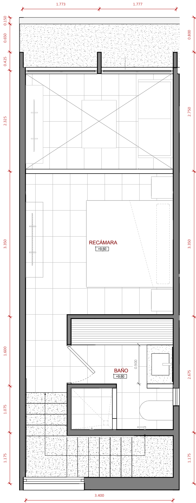
NIVEL 4 +9.60 ESCALA 1 : 50
