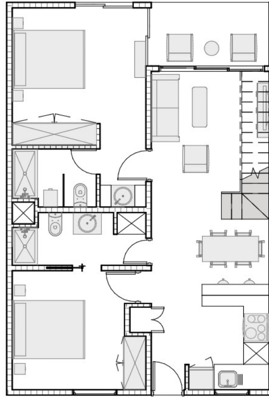
Apartamento 2 habitaciones: 73.00 m 2 Balcón: 7.00 m 2
