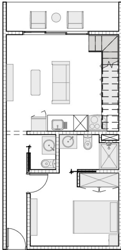
Apartamento 1 habitación: 50.00 m 2 Balcón: 6.30 m 2
