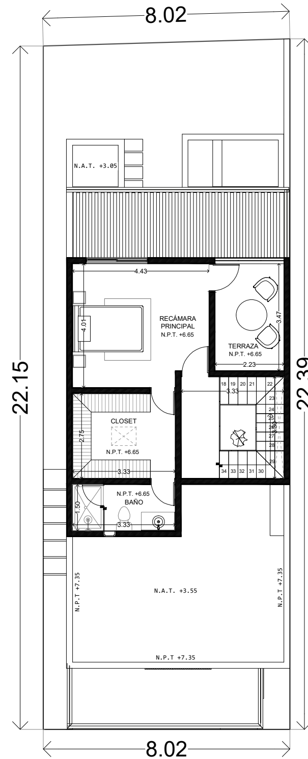
SEGUNDO NIVEL
