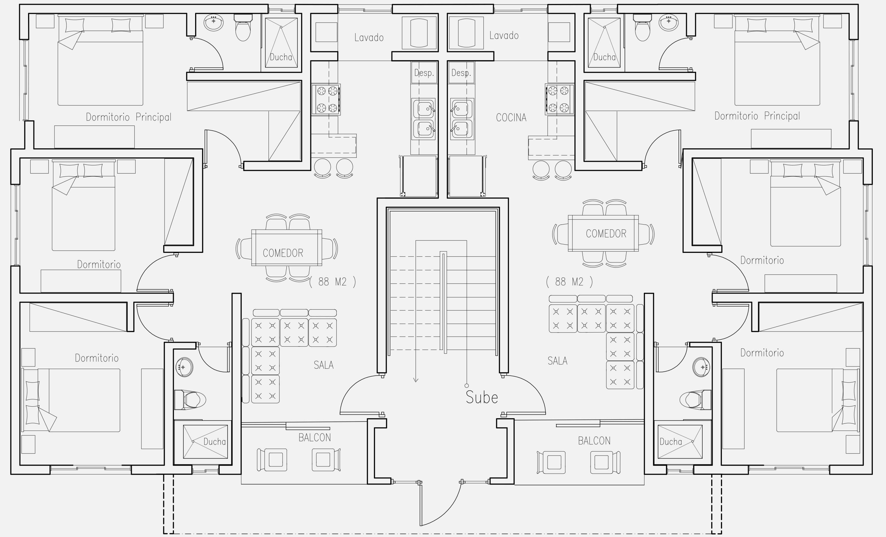
PRIMER NIVEL
