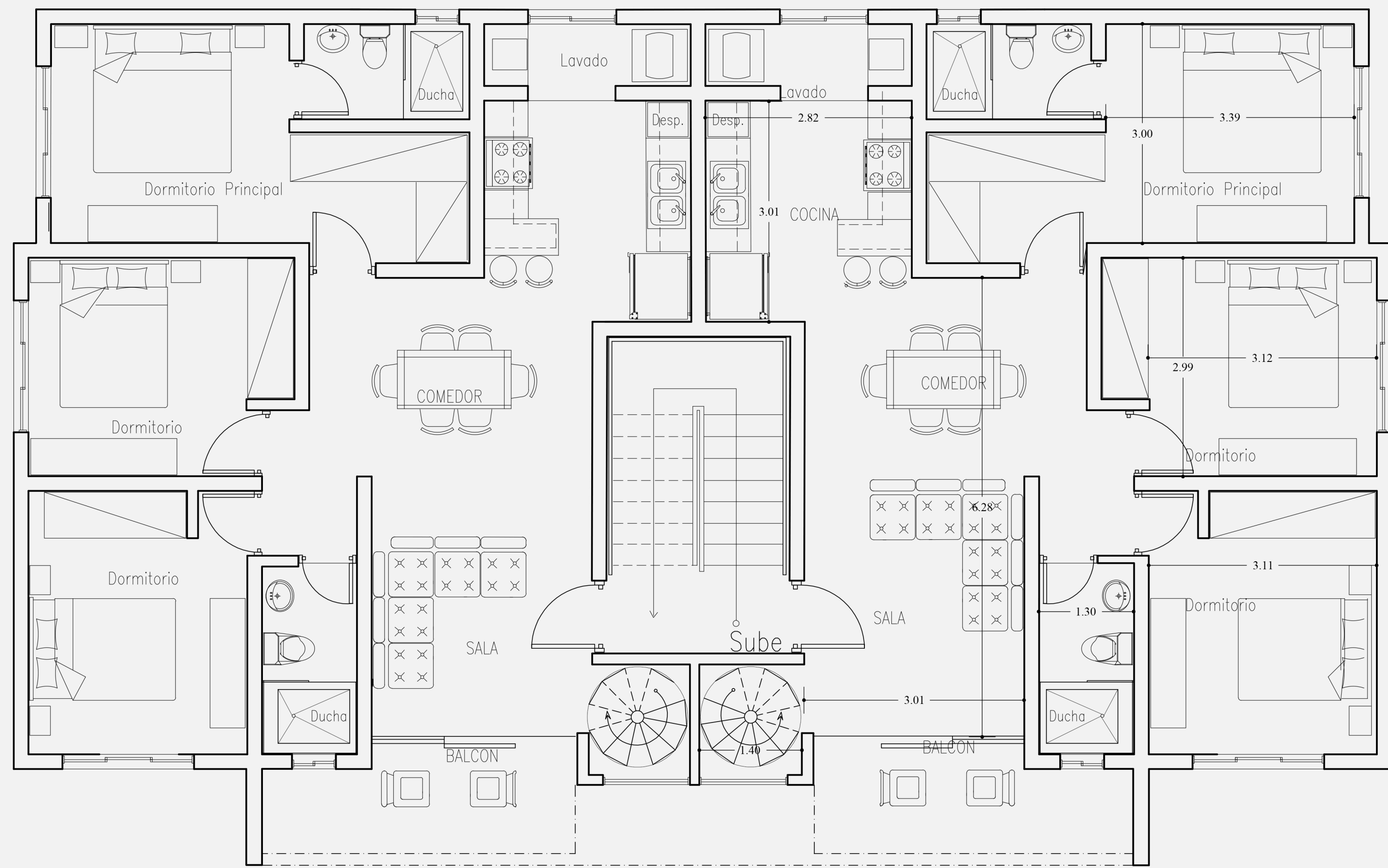
TERCER NIVEL
