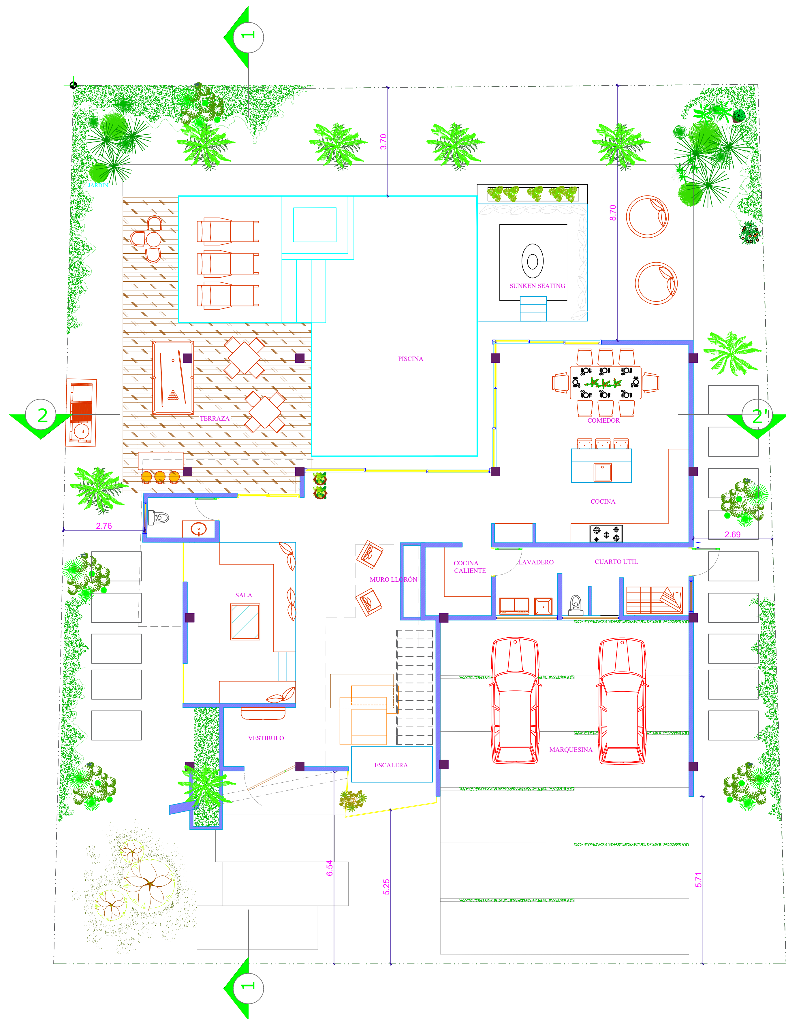
PLANTA ARQUITECTONICA 1ER NIVEL
