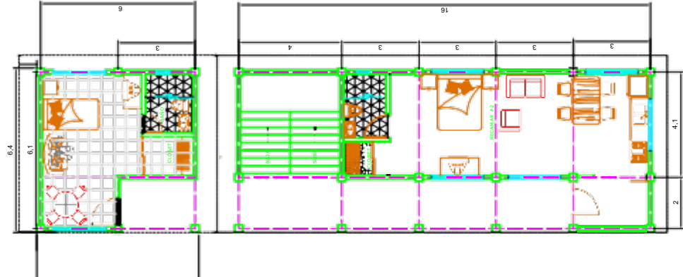
PLANTA ARQUITECTONICA NIVEL 2 ESC : 1 : 100
