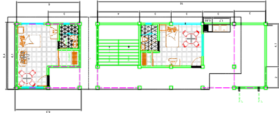
PLANTA ARQUITECTONICA NIVEL 3 ESC : 1 : 100
