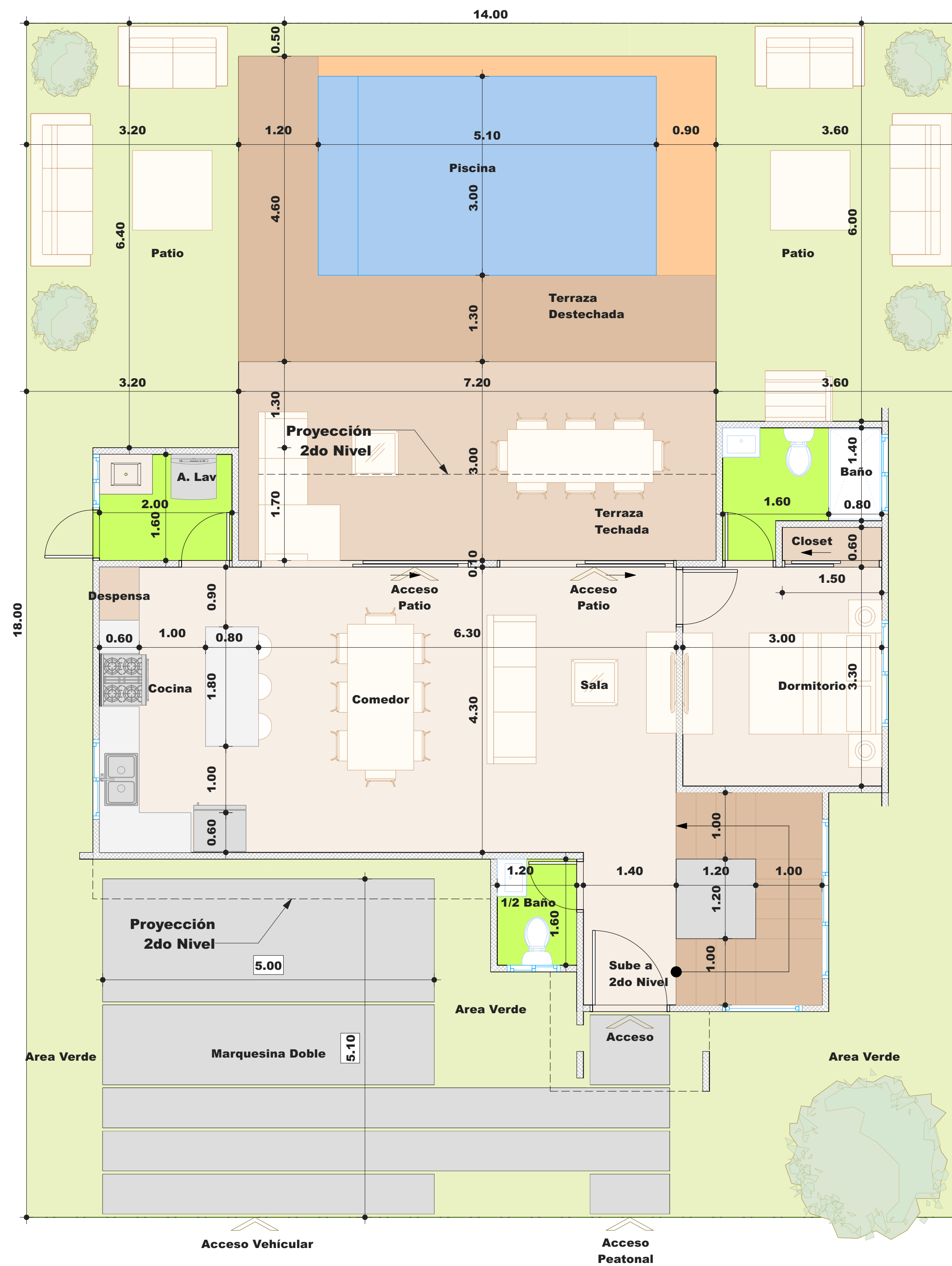
5 Planta Arq. 1er Nivel (Villa Tipo U) Scale: 1:50
