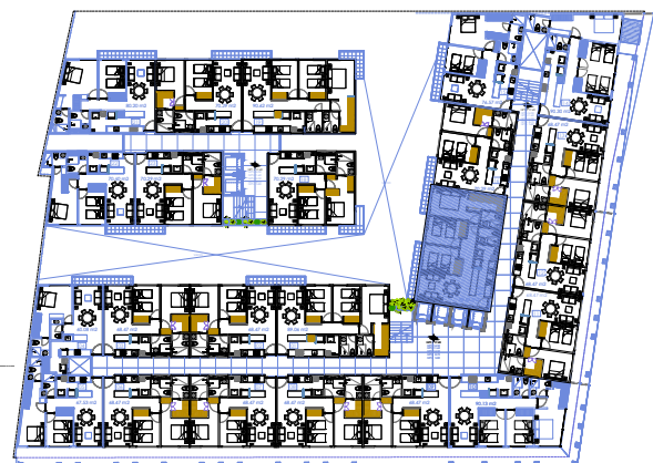
UBICACION DEPTOS. PLANTA TIPO T-3R SIN ESC. ACOT. M
