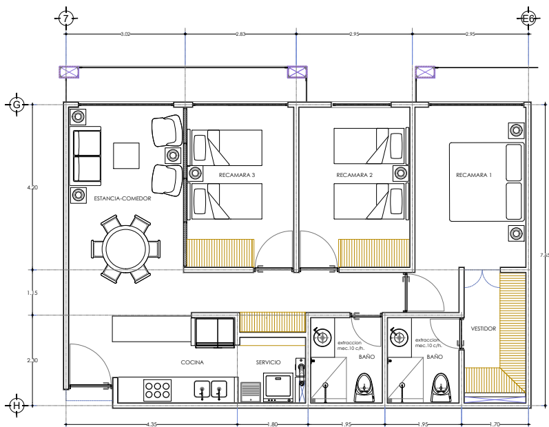
PLANTA ARQUITECTONICA T-3R ESC. 1:125 ACOT. M
