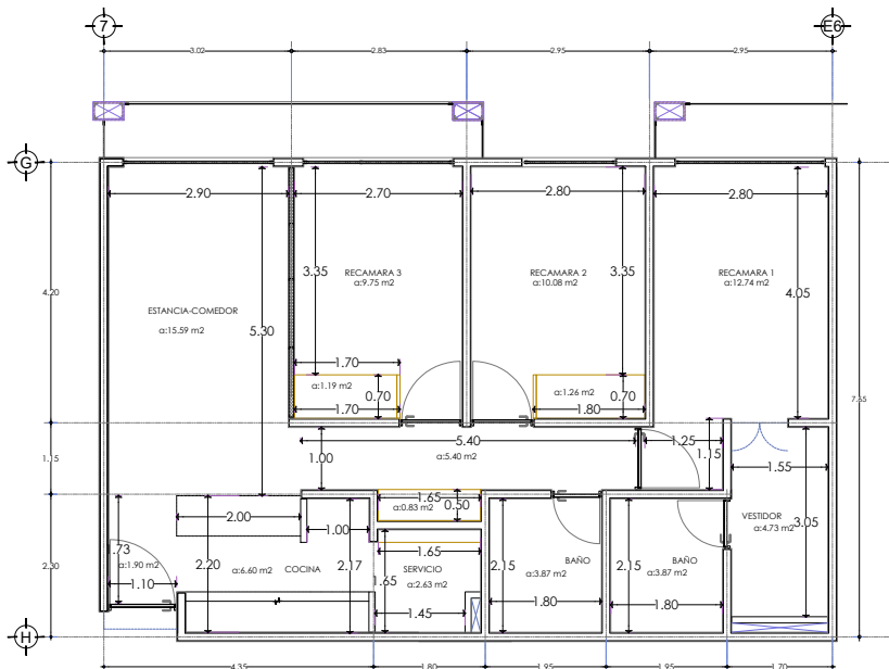
AREAS T-3R ESC. 1:125 ACOT. M
