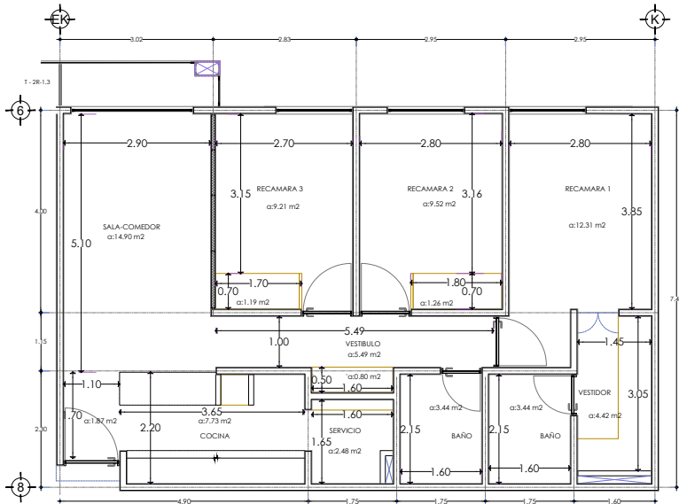
AREAS T-3R1.1 ESC. 1:125 ACOT. M
