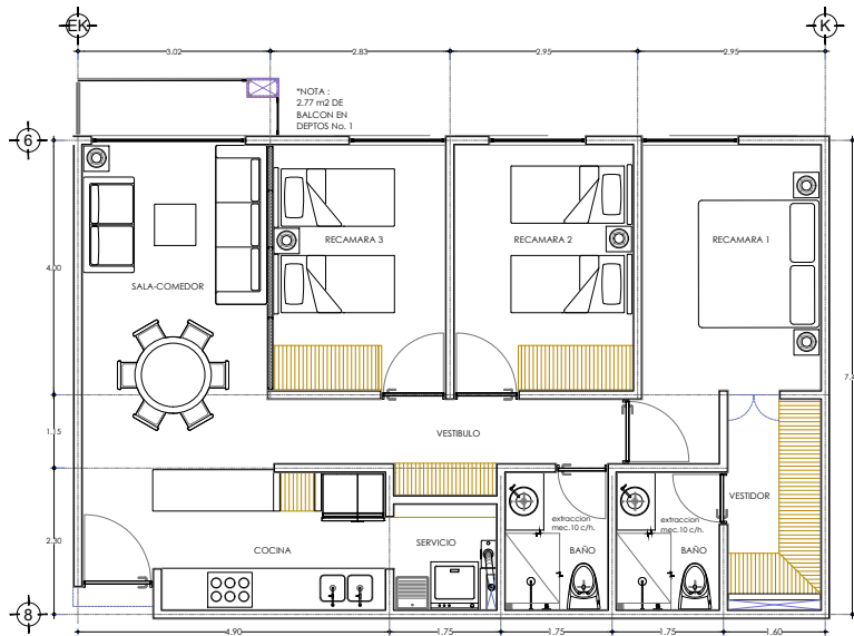
PLANTA ARQUITECTONICA T-3R1.1 ESC. 1:125 ACOT. M
