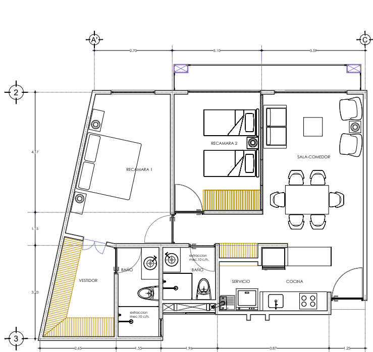
PLANTA ARQUITECTONICA TIPO T-2R ESC. 1:125 ACOT. M
