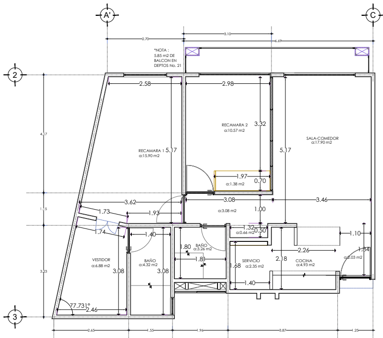
AREAS T-2R ESC. 1:125 ACOT. M
