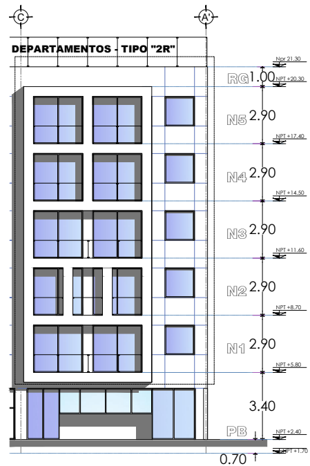
ELEVACION DEPTO. TIPO T-2R ESC. 1:25 ACOT. M
