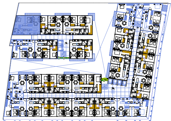
UBICACION DEPTOS. PLANTA TIPO T-2R SIN ESC. ACOT. M
