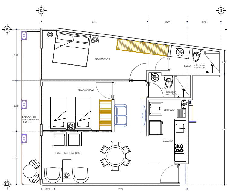
PLANTA ARQUITECTONICA T-2R-1.4 ESC. 1:125 ACOT. M
