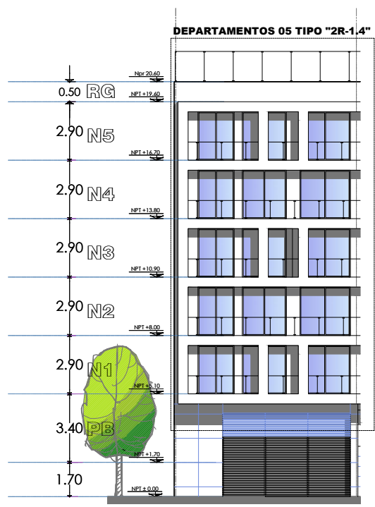
ELEVACION DEPTOS 05 T-2R-1.4 ESC. 1:25 ACOT. M
