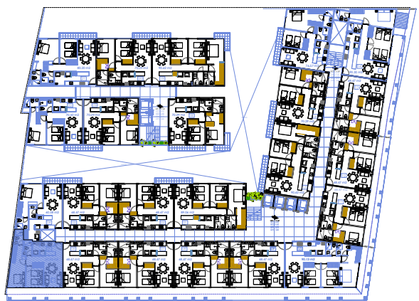
UBICACION DEPTOS. PLANTA TIPO T-2R-1.4 SIN ESC. ACOT. M
