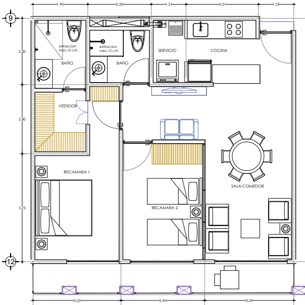
PLANTA ARQUITECTONICA T-2R-1.3A ESC. 1:125 ACOT. M
