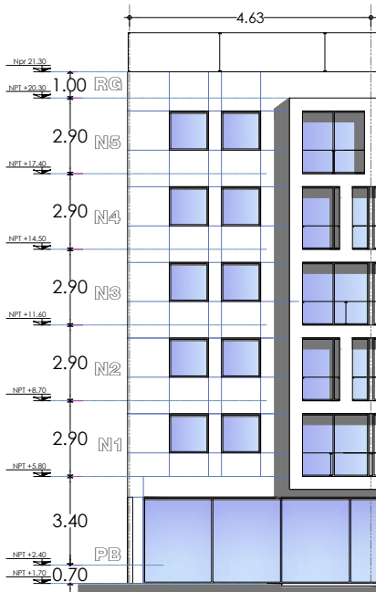
ELEVACION DEPARTAMENTOS T-2R1.1 ESC. 1:25 ACOT. M
