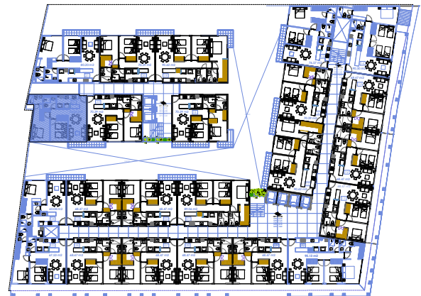
UBICACION DEPTOS. PLANTA TIPO T-2R1.1 SIN ESC. ACOT. M
