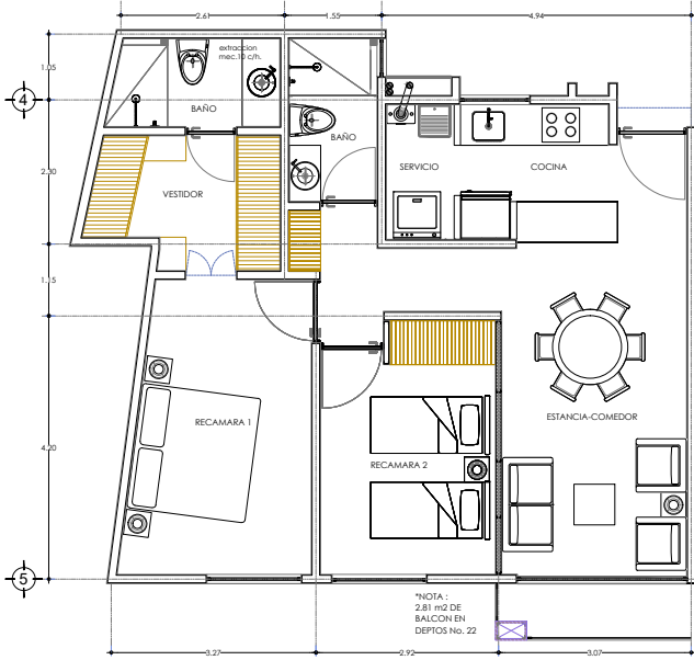
PLANTA ARQUITECTONICA T-2R1.1 ESC. 1:125 ACOT. M
