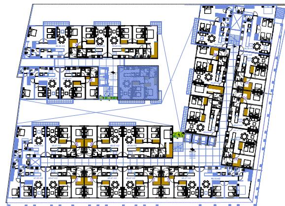
UBICACION DEPTOS. PLANTA TIPO T-2R-1.2' SIN ESC. ACOT. M
