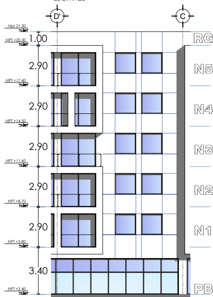
ELEVACION DEPTOS. No. 20 T-2R1.2 ESC. 1:25 ACOT. M
