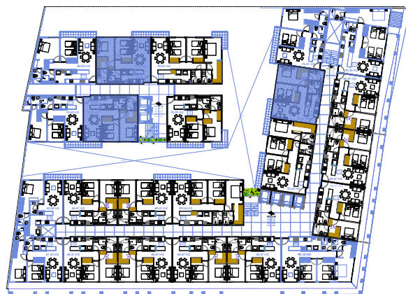
UBICACION DEPTOS. PLANTA TIPO T-2R1.2 SIN ESC. ACOT. M
