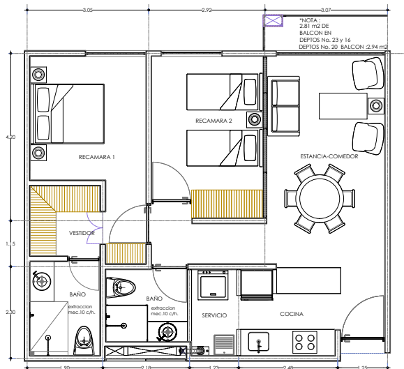
PLANTA ARQUITECTONICA T-2R1.2 ESC. 1:125 ACOT. M
