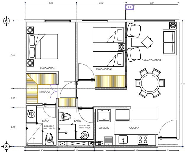
PLANTA ARQUITECTONICA T-2R-1.3 ESC. 1:125 ACOT. M
