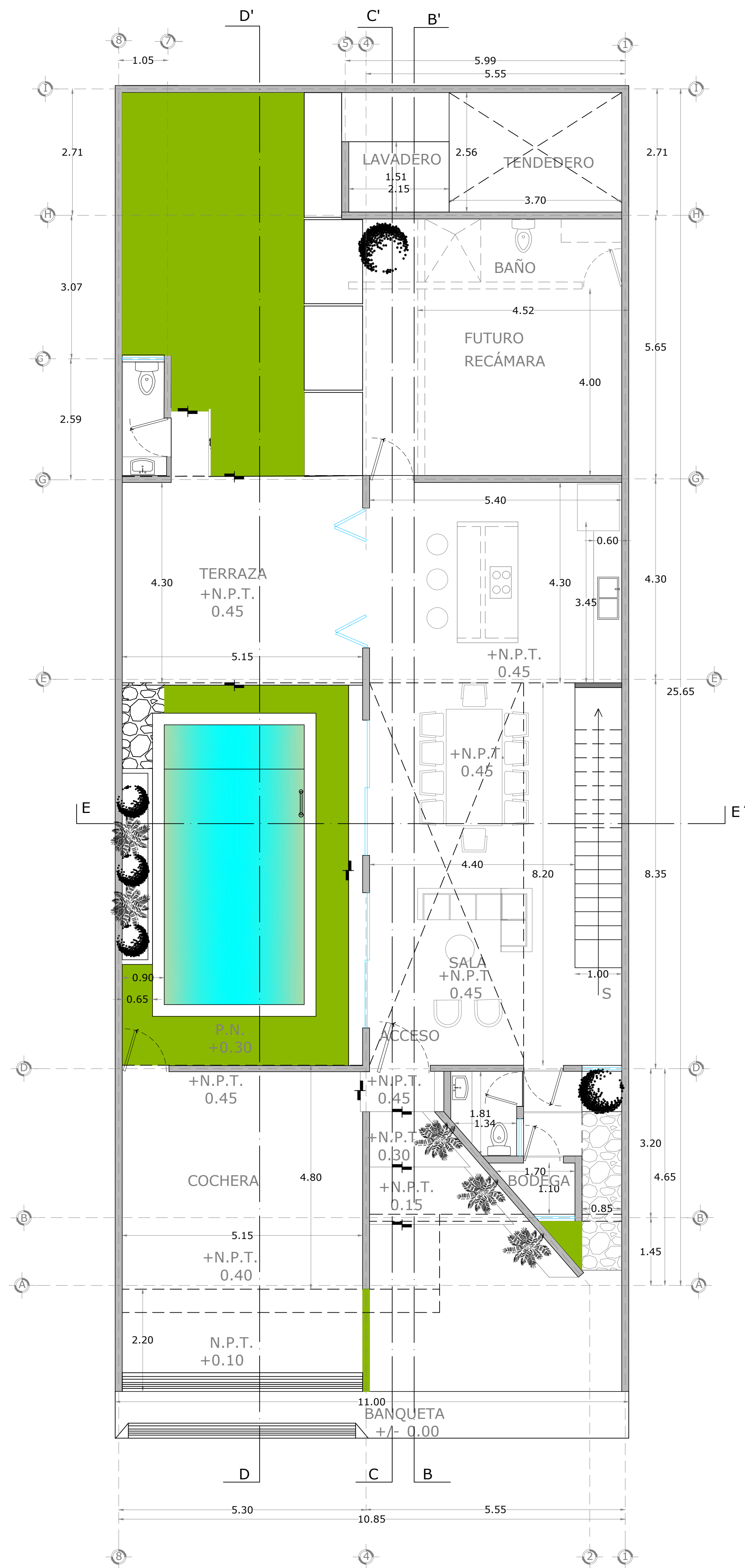
PLANTA BAJA
