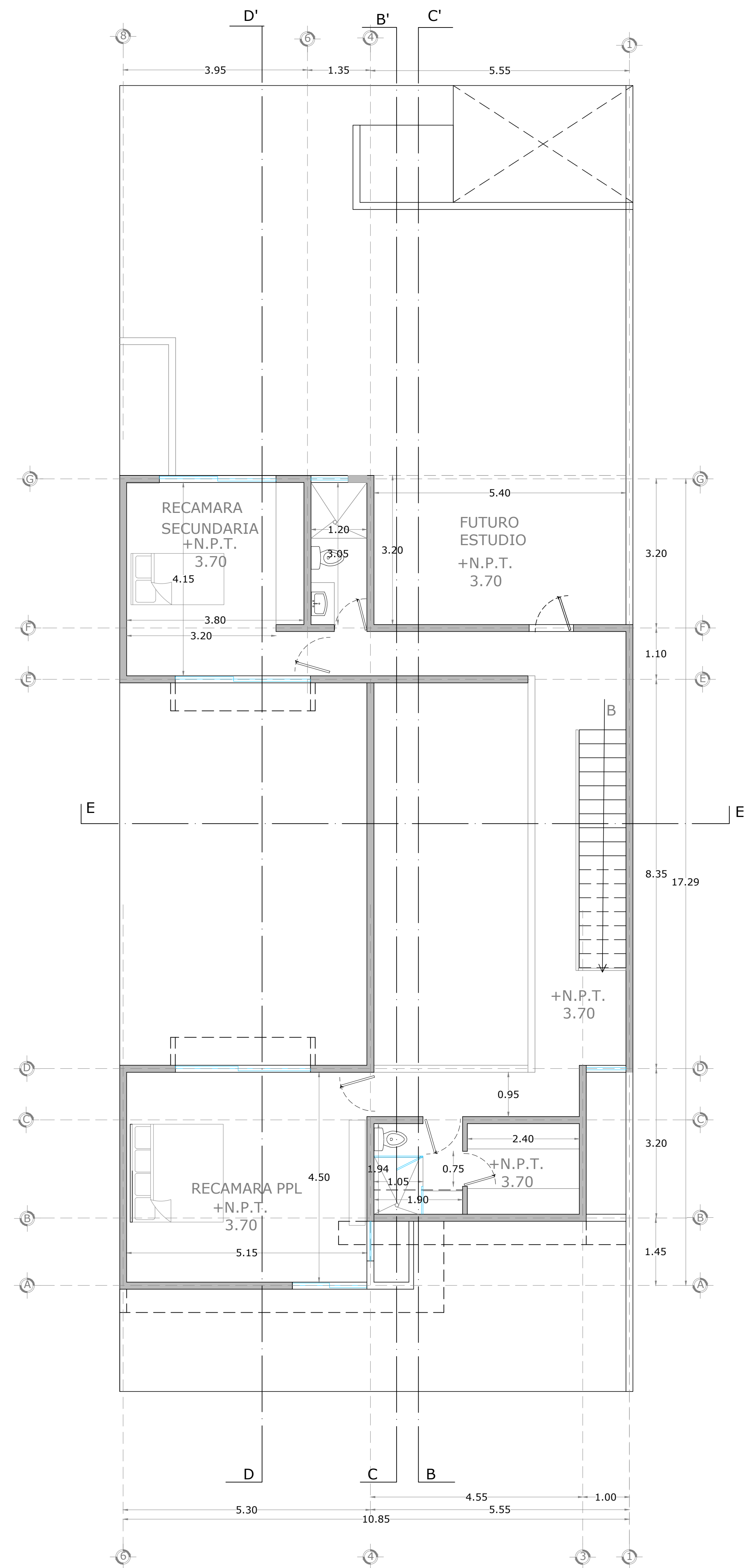
PLANTA ALTA
